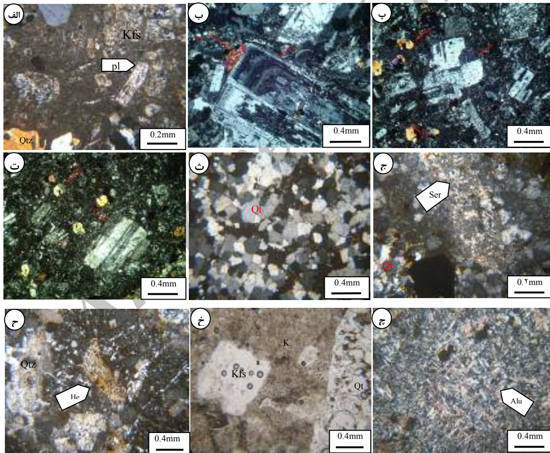
شکل ۵ الف- تصویر میکروسکوپی از ریولیت‌های منطقه (XPL) ب- تصویر میکروسکوپی از کوارتز مونزودیوریت پورفیری (XPL) پ- تصویر میکروسکوپی از پیروکسن هورنبلند دیوریت پورفیری، کانی هورنبلند به کلریت دگرسان شده است. (XPL) ت- تصویر میکروسکوپی از آندزیت (XPL) ث- تصویر میکروسکوپی از رگه کوارتزی (XPL) ج- تصویر میکروسکوپی از دگرسانی آرژلیک-کوارتز-سرسیت-پیریت (XPL) ح- تصویر میکروسکوپی از دگرسانی سیلیس-آرژلیک-زمینه آرژیلی شده است و پیریت نیز به اکسیدهای آهن تبدیل شده است (XPL) خ- تصویر میکروسکوپی از دگرسانی سیلیس-آرژلیک (PL) چ- تصویر میکروسکوپی از دگرسانی آرژلیک پیشرفته (XPL) علائم اختصاری [۲۲] و Ser برای سرسیت، Alu برای آلونیت استفاده شده است.
