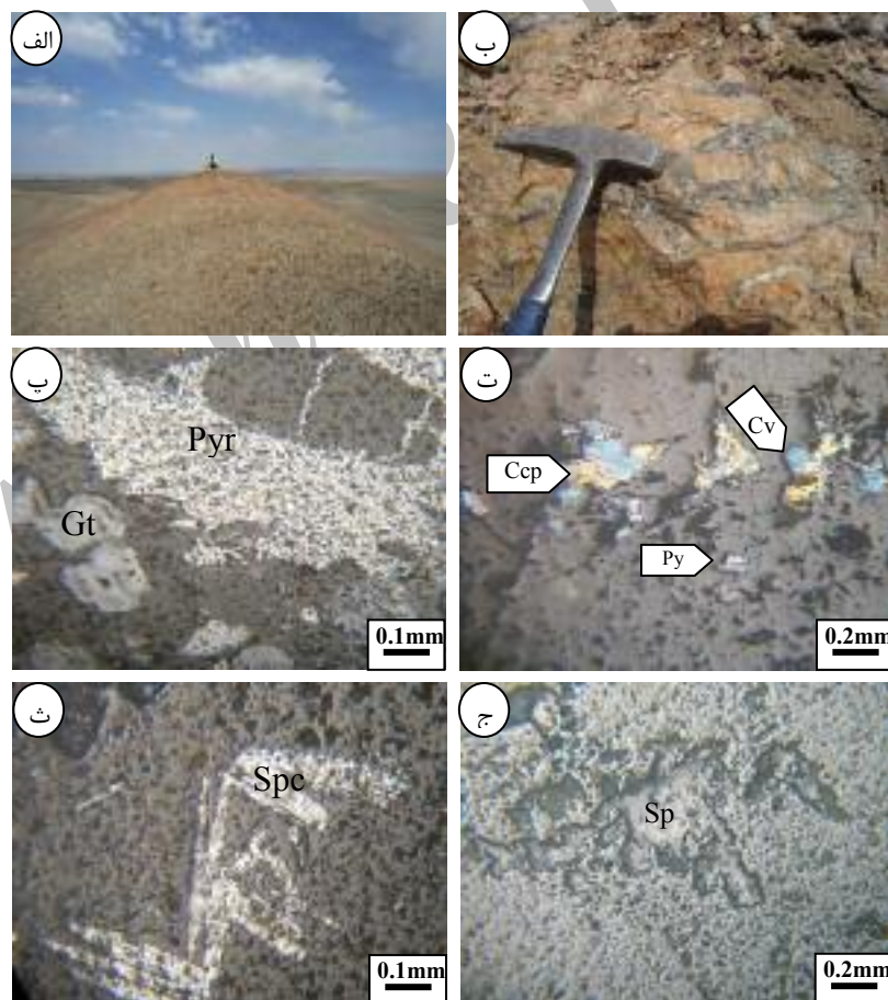
شکل ۷ الف- کلاhek گوسان (دید به سمت شمال) ب- کانی‌سازی پیرولوویت و گوتیت در زمینه‌ی برش گرمایی پ- کانی‌زایی گوتیت و پیرولوویت ت-کانی‌سازی کالکوپیریت، کولیت و پیریت در رگه‌های کوارتز-کربنات ث- کانی اسپیکیولاریت ج- کانی اسفالریت × علائم اختصاری بر اساس [۲۲] و Spc برای اسپیکیولاریت استفاده شده است.
