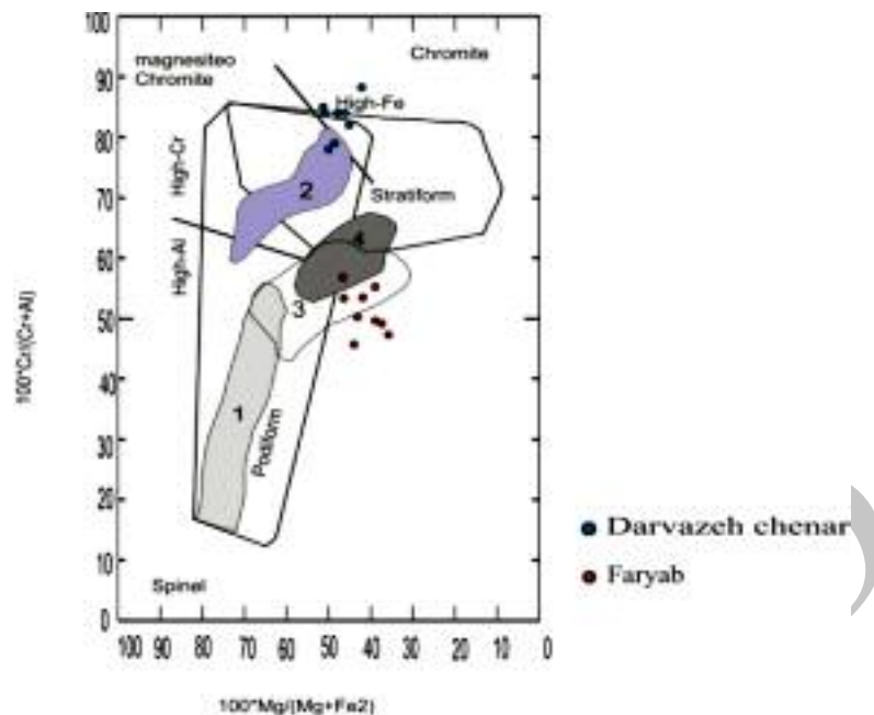
شکل ۱۰ ترکیب کرومیت‌های فاریاب و دروازه چنار در نمودار Cr# نسبت به Mg# و مقایسه‌ی کرومیت‌های این مناطق با پریدوتیت‌های عمیق (۱)، افیولیت‌های تروُدوس (۲)، غلاف‌های کوچک و عمیق هسی (۳)، و کرومیت‌های انبان‌های پوسته بالایی افیولیت عمان (۴).
