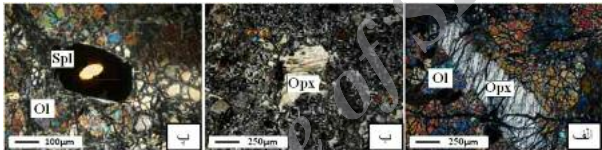
شکل ۲ مقطع نازک از پریدوتیت‌های بررسی‌های نیریز، الف) دونیت حاوی اولیوین و پیروکسن (XPI، ب) دونیت سرپانتینی شده حاوی ارتوپروکسن (XPL، پ) دونیت حاوی اولیوین و اسپینل کرومیت (XPL)
