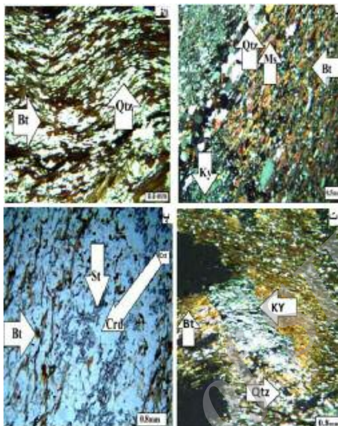
شکل ۲ تصاویر میکروسکوپی از نمونه‌های متاپلیتی منطقه الف- شیسوزیته غالب در متاپلیت‌ها. ب- کانی‌های موجود در متاپلیت‌ها را نشان می‌دهد. پ- پورفایروپلاست‌های استارولیت و کردیریت را به صورت تشکیل دوگانه با هم نشان می‌دهد. ت- پورفایروپلاست کیانیت در نمونه‌های متاپلیتی را مشخص می‌کند. تصاویر الف و پ در حالت PPL و ب و ت در حالت XPL تهیه شده‌اند.
