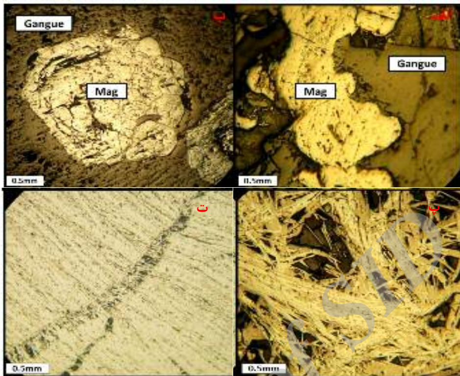
شکل ۱۷ الف) حضور مگنتیت (Mag) به صورت بی‌شکل در واحدهای میزبان کانی‌زایی (نور بازتابی با بزرگنمایی 100X)، ب) وجود مگنتیت شکل‌دار در برش سیلیسی شده (نور بازتابی با بزرگنمایی 50X)، پ و ت) تأثیر فرآیندهای Mushketovitzation بر هماتیت و تبدیل آن به مگنتیت (نور بازتابی با بزرگنمایی 100X).
