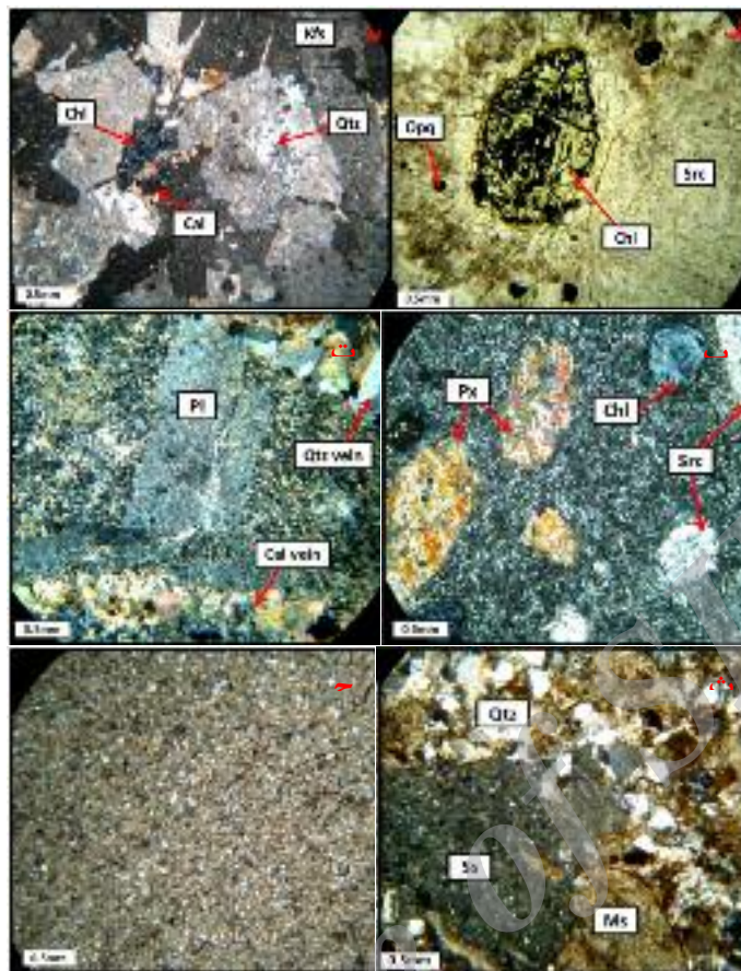
شکل ۹ الف) دگرسانی کامل پلاژیوکلاز به سریسیت (Src) و عملکرد دگرسانی گرمایی و رشد کانی‌های کدر (Opq) در رخ‌ها و شکستگی‌های الیون و دگرسانی آن به کلریت (Chl) در مونوسینیت، ب) وجود بافت دانه ای و درشت بلورهای فلدسپار پتاسیم (Kfs) در واحدهای سینیتی منطقه و نیز پرشدگی فضای خالی به وسیله کانی‌های کوارتز (Qtz) و کلسیت (Cal)، ج) پرشدگی فضاهای خالی سنگ‌های بازالتی به ویژه با کانی کلسیت و تشکیل بافت بادامکی و تأثیر دگرسانی و رشد کانی‌های کدر اطراف کلریت‌ها در واحدهای بازالت پورفیری. د) درشت بلورهای پلاژیوکلاز در حال تجزیه به کانی‌های سریسیت همراه با رگچه‌های کلسیتی و سیلیسی در سنگ‌های آندزیت پورفیری، ه) حضور کوارتز، سیلتستون (Pl) و گل سنگ (Ms) در کنگلومرا و و) واحدهای سیلتستون منطقه‌ی مورد بررسی که دارای بافت ریزدانه است (همه تصاویر در نور قطبیده متقاطع با بزرگنمایی 40X تهیه شده‌اند).
