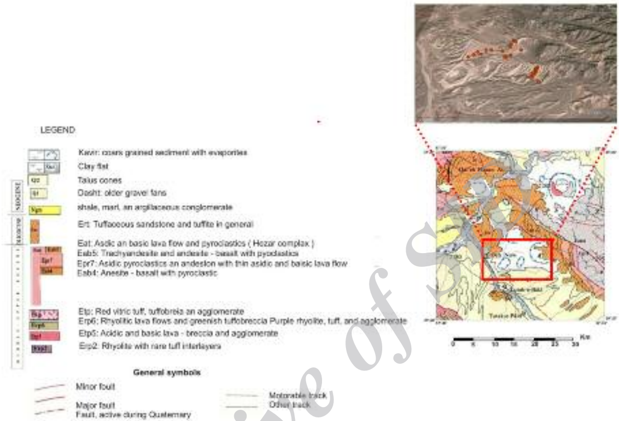
شکل ۱ نقشه‌ی زمین‌شناسی منطقه‌ی مورد بررسی [۶] در شکل مشخص شده است.
