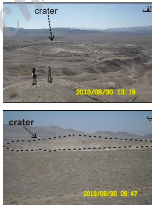
شکل ۲ کراترهای منطقه توتک در راین.
