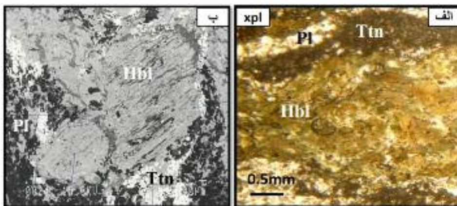
شکل ۹ الف) تصویر میکروسکوپی هورنبلند (Hbl) سبز مایل به قهوه‌ای، تیتانیت (Ti) و پلاژیوکلاز از شبه‌بازی‌های ده‌سلم در نمونه‌ی Sb1، ب) تصویر BSE هورنبلند، تیتانیت و پلاژیوکلاز آنالیز شده در نمونه‌ی Sb1 با مقیاس 100. µm
