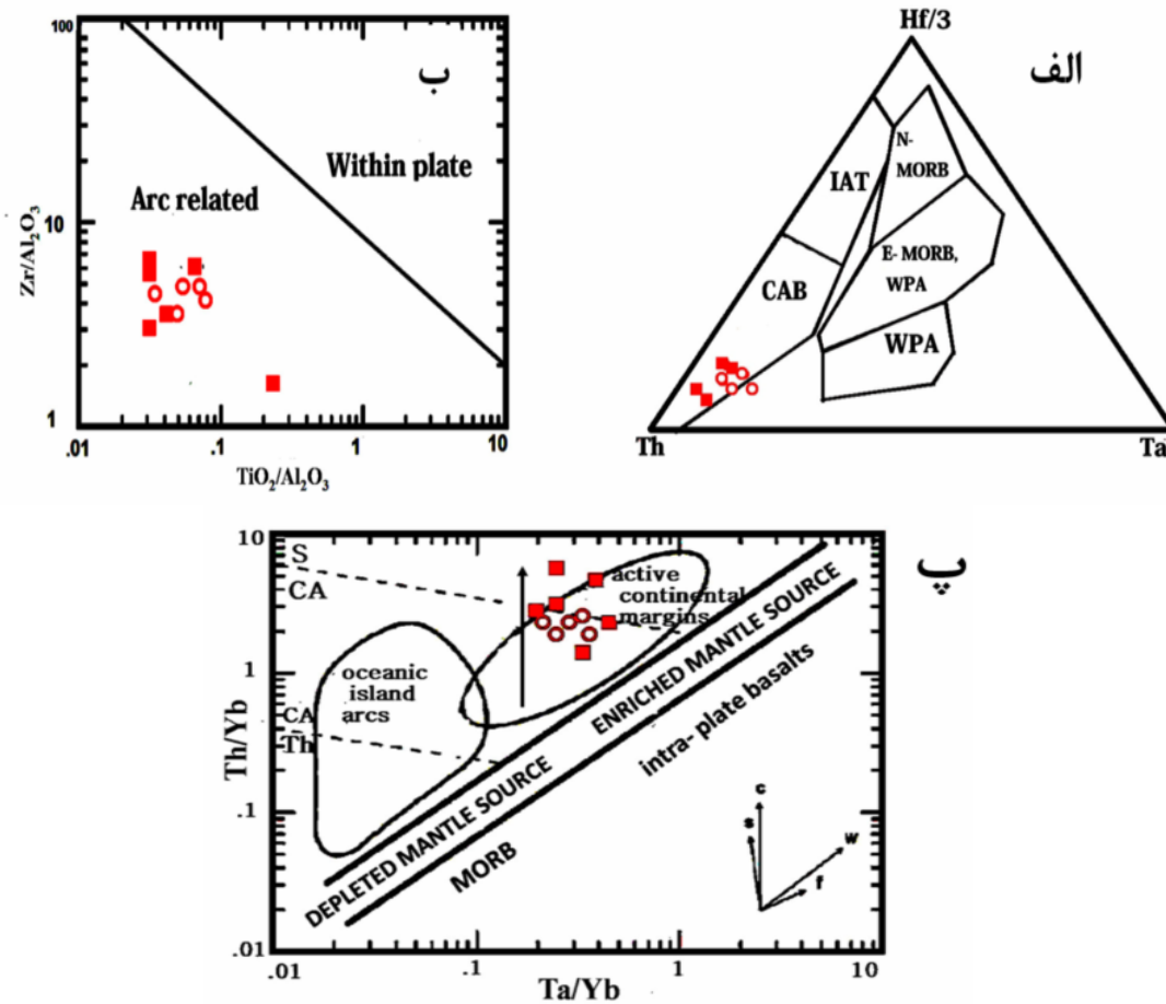
شکل ۸ الف) تعیین محیط‌های زمین‌ساختی سنگ‌های آتشفشانی مورد بررسی با استفاده از نمودار Hf/3 - Th - Ta [۲۱]. ب) جدایش گستره-های آتشفشانی از درو صفح‌های با استفاده از نمودار Zr/Al_2O_3 در مقابل TiO_2/Al_2O_3 [۲۲]. پ) محیط تکتونیکی سنگ‌های منطقه و تفکیک کمان ماگمایی حاشیه فعال قاره‌ای از نوع کمان‌ها جزیره‌ای براساس تغییرات Th/Yb در برابر Ta/Yb [۲۳].
