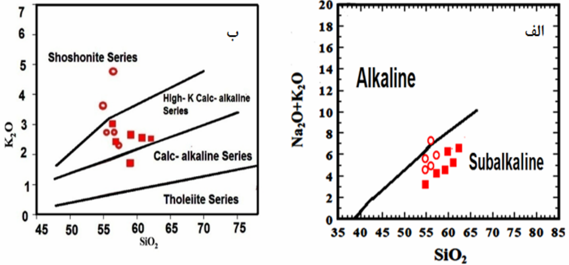
شکل ۷ تعیین سری ماگمایی سنگ‌های آتشفشانی منطقه‌ی ابری با استفاده از نمودارهای ارائه شده: الف) نمودار Na_2O + K_2O در مقابل به SiO_2 [۱۸]. ب) نمودار K_2O در مقابل SiO_2 [۱۹].
