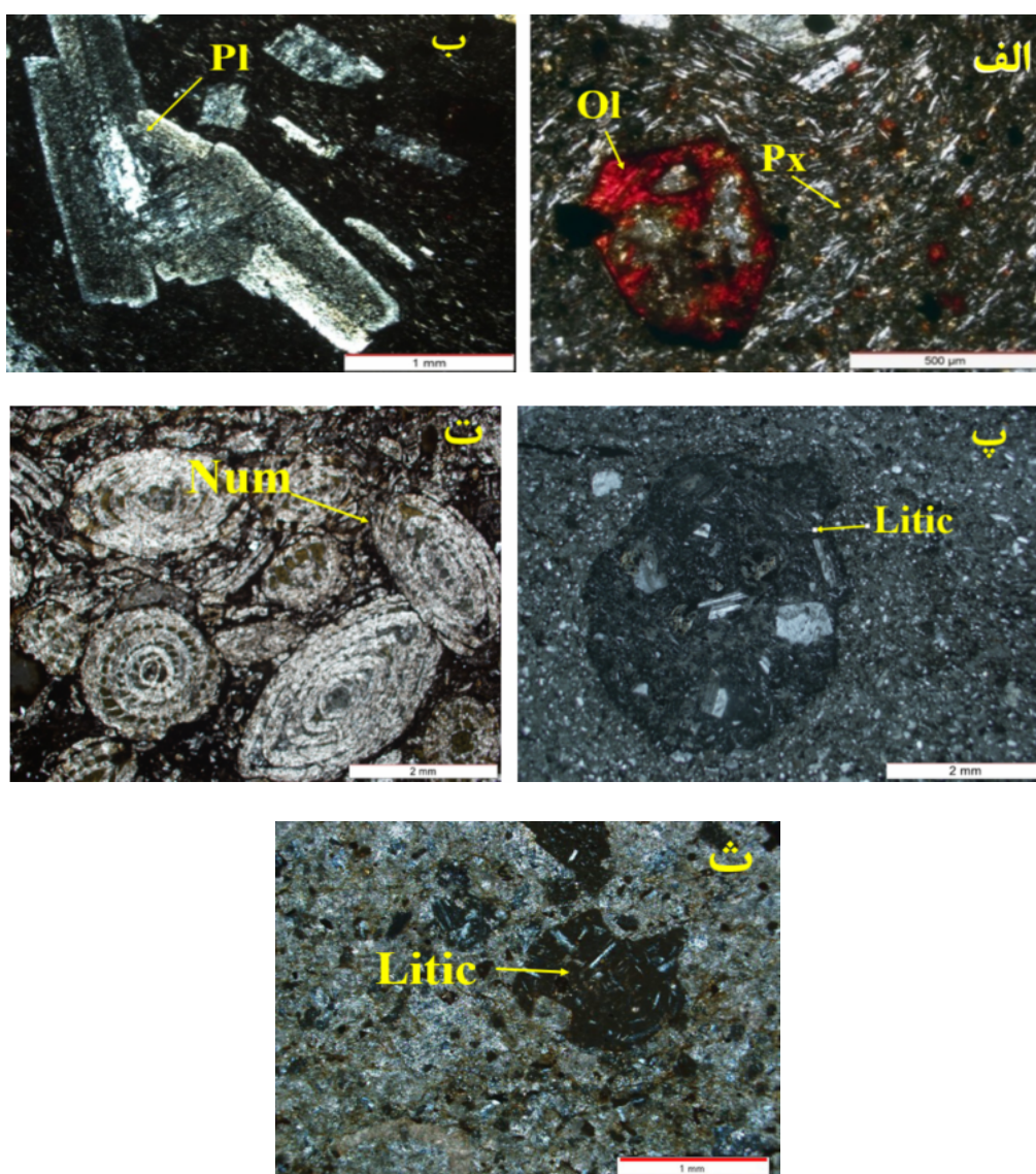
شکل ۴ الف) پیروکسن و الیوین ایدنگزیتی شده، در زمینه دانهریز و میکرولیتی آندزیت بازال‌ها. ب) پلاژیوکلازها با بافت‌های غربالی و گلومروپورفیری در واحد آندزیتی پ) کریستال توف و لیتیک توف با ترکیب آندزیت. ت) حضور فسیل نومولیت در داخل واحد آهک. ث) حضور قطعات سنگی با ترکیب آندزیت در داخل واحد آهک. Px: پیروکسن، Ol: الیوین، Litic: قطعات سنگی، Num: فسیل نومولیت.
