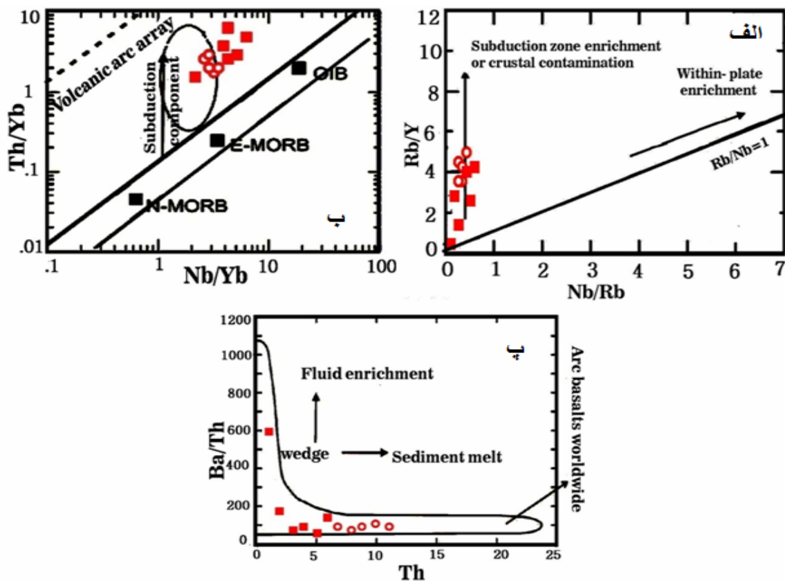
شکل ۹ الف) موقعیت سنگ‌های منطقه‌ی مورد بررسی در نمودار Rb/Y در برابر Nb/Rb [۲۶]. ب) نمودار Th/Yb در برابر Nb/Yb [۲۷]. پ) تعیین نقش رسوبات فرورنده با استفاده از نمودار Ba/Th در برابر Th [۳۰].
