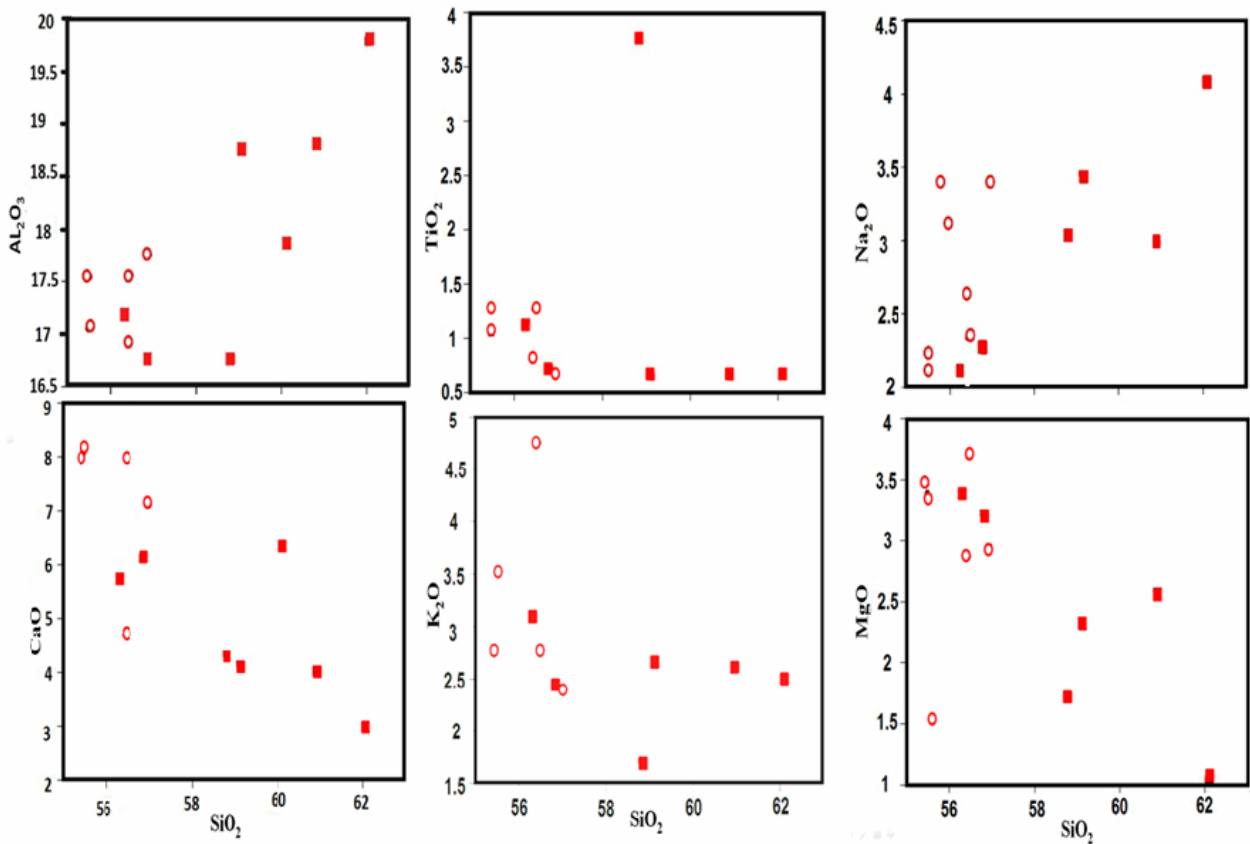
شکل ۶ تغییرات مقادیر اکسیدهای اصلی در برابر درصد وزنی SiO_2 در سنگ‌های آتشفشانی دربرگیرنده کانسار مس ابری [۱۴]. با افزایش SiO_2 میزان Na_2O ، Al_2O_3 و CaO کاهش و P_2O_5 ، FeO ، MgO افزایش نشان می‌دهند.
