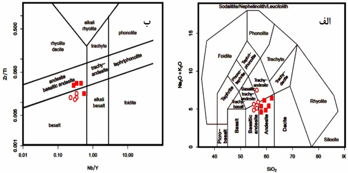
شکل ۵ الف) موقعیت سنگ‌های آتشفشانی محدوده کانسار مس ابری در نمودار SiO_2 در برابر (Na_2O+K_2O) ، [۱۲] نمونه‌ها در گستره آندزیت، تراکی آندزیت و آندزیت بازالتی قرار می‌گیرند. ب) موقعیت آنها در نمودار Zr/Ti نسبت به Nb/Y [۱۳]. علامت اختصاری عبارتند از:
