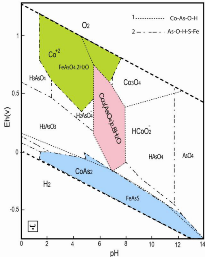
شکل ۵ الف) مقاطع میکروسکوپی که در آن دگرسانی آرسنوپیریت به اسکوردیت و اریترایت دیده می‌شود. ب) طرحواره از مراحل پیشرفت دگرسانی آرسنوپیریت و تولید فراورده‌های ثانویه. پ) نمودار Eh-pH برای سیستم Co-As-O-H (محدوده خط چین شماره ۱) و سیستم AS-O-H-S-Fe (محدوده خط چین شماره ۲) که در دمای 25°C و فشار یک بار رسم شده است. غلظت ترکیبات \sum Co , \sum Fe , \sum S , \sum As همه در 10^{-3} M ثابت نگه داشته شده است [۲۱-۱۸]. ناحیه‌های رنگی نشان دهنده حوزه پایداری کانی‌های آرسنوپیریت، اسکوردیت و اریترایت است.
