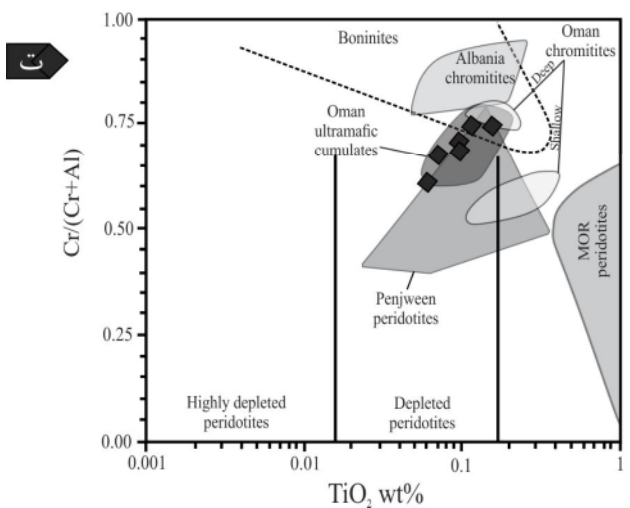
شکل ۶ الف: نمودار Al_2O_3 نسبت به TiO_2 کروم اسپینل پریدوتیت‌های مجموعه افیولیتی کرمانشاه. ( میدان‌ها از مراجع [۳۵ و ۱۹]). ب: نمودار Cr_2O_3 نسبت به Al_2O_3 کروم اسپینل پریدوتیت‌های مجموعه افیولیتی کرمانشاه. پ: نمودار Al_2O_3 نسبت به TiO_2 کروم اسپینل (میدان‌های بونینیت از [۲۲]، بونینیت ترودوس از [۴۱]، بونینیت تدفورد از [۴۲]، و MORB از [۴۳])، ت: نمودار Cr\# نسبت به TiO_2 کروم اسپینل پریدوتیت‌ها (میدان‌های پریدوتیت آیسال از [۲۰]، کوموله‌های عمان از [۲۳]، کرومیت‌های عمان از [۲۴] و پریدوتیت‌های پنجوین از [۶] برای مقایسه آورده شده‌اند). علائم همانند شکل ۵.
