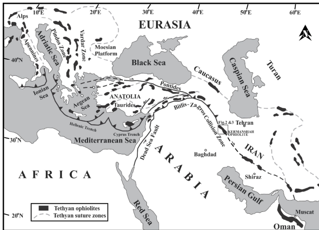
شکل ۱ پراکندگی افیولیت‌های تیتسی در مناطق جوش خورده‌ی سیستم کوهزایی آلپ-همالیا، برگرفته از مرجع [۱] با اندکی تغییرات.
