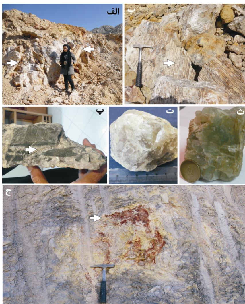
شکل ۴ الف: رگه‌های فلوریت و کوارتز در جنوب منطقه کوه سفید، ب: نمایی از رگه‌های کانی‌سازی کوارتز، پ: رگه‌های فلوریت-کوارتز (جنوب منطقه مورد بررسی)، ت: فلوریت سفید، ث: فلوریت سبز، ج: لیمونیت و هماتیت (جنوب منطقه مورد بررسی).
