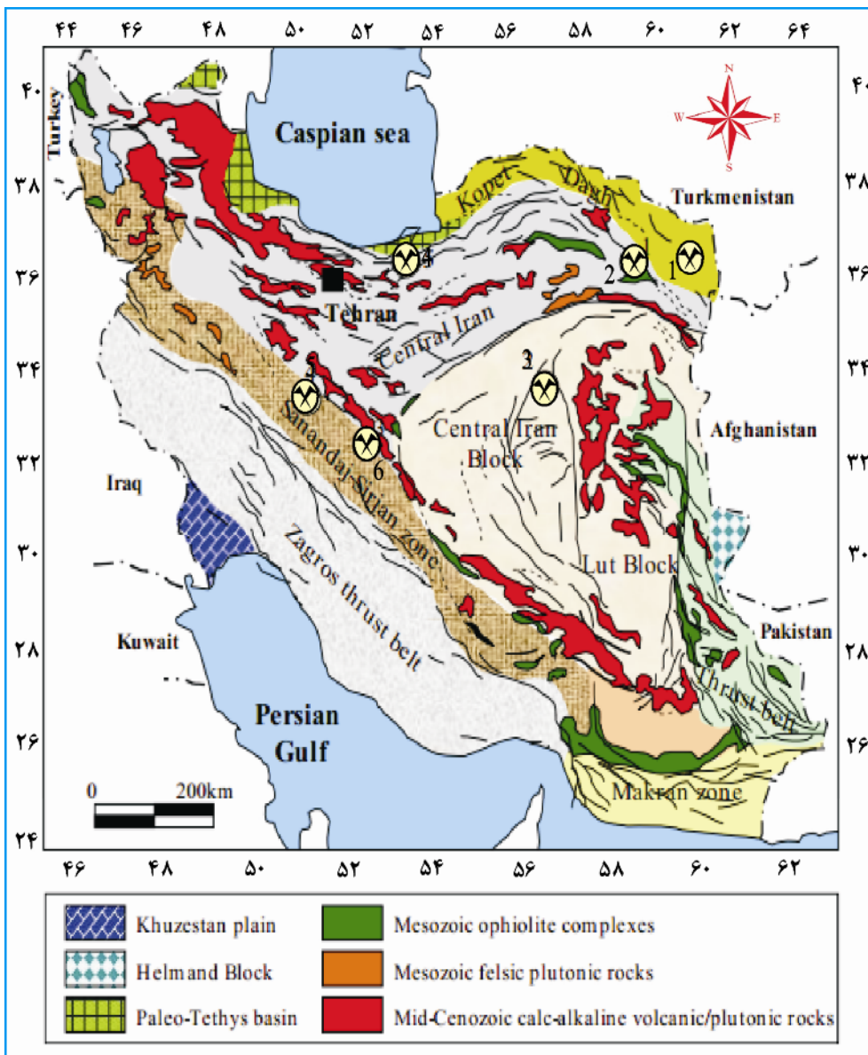
شکل ۱ موقعیت برخی از کانسارهای فعال فلوریت در نقشه زمین‌شناسی ایران [۳]. این معادن به ترتیب شامل ۱- فلوریت سفیدکوه، ۲- فلوریت جویمند گناباد، ۳- فلوریت کمرمهدی طبس، ۴- فلوریت پیناوند و کمشچه اصفهان، ۵- کمربند فلوریت محلات- دلیجان و ۶- کمربند فلوریت کیاسر- پل سفید (شامل منطقه سوادکوه) است.
