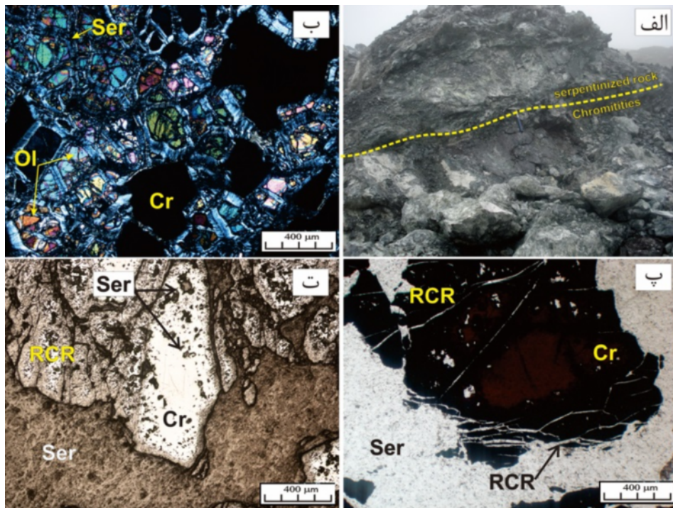
شکل ۲ الف) تصویر صحرایی کرومیت‌های Cr بالا احاطه شده توسط پریدوتیت سرپانتینی شده در بخش غربی افیولیت خوی، ب) الیون (Ol) و سرپانتین (Ser) در فضای بین دانه‌های کروم اسپینل (Cr)، پ) کروم اسپینل (Cr) به رنگ قهوه‌ای روشن در نور طبیعی عبوری (PPL) و کناره تیره (RCR) به دلیل حضور فروکرومیت از کرومیت‌های Al بالا در بخش شرقی افیولیت خوی، و ت) میانبرهای پر شده با سرپانتین (Ser) در کروم اسپینل.
