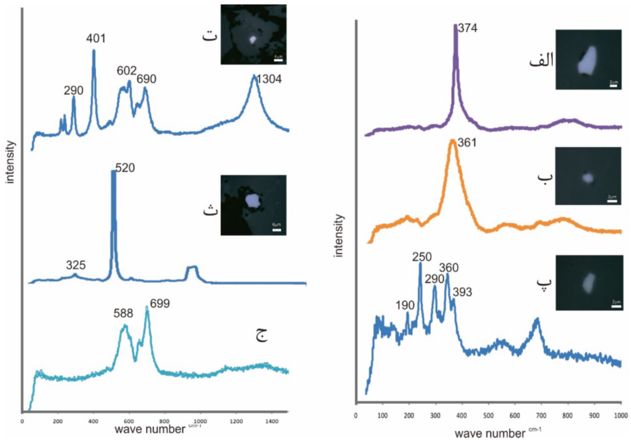
شکل ۶ الف و ب) طیف‌های رامان برای لاوریت با Ru>Os و پ) ایرارسیت غنی از Rh که به صورت میانبار در کروم اسپینل‌های غنی از Cr در بخش غربی افیولیت خوی قرار دارند، ت) طیف رامان مربوط به هماتیت و ث) آهن خالص (؟) در محل شکستگی‌های کروم اسپینل، ج) طیف رامان مربوط به کروم اسپینل میزبان، به همراه تصویر میکروسکوپی تهیه شده توسط طیف سنج رامان.
