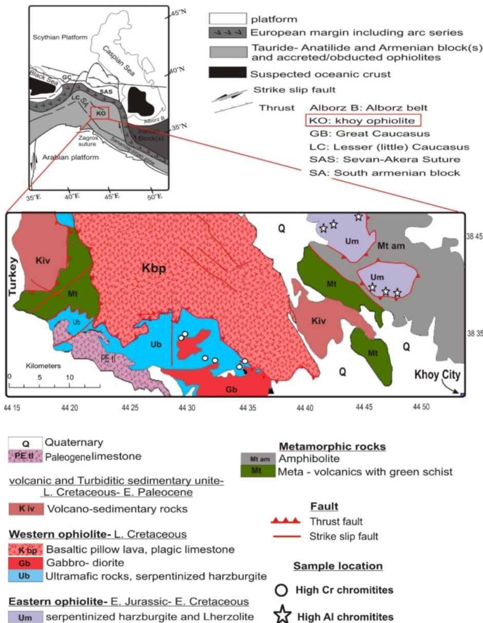
شکل ۱ نقشه زمین‌شناسی ساده شده از منطقه مورد بررسی به همراه محل تقریبی نمونه‌برداری کرومیت‌ها در بخش غربی افیولیت و بخش شرقی افیولیت خوی به همراه نقشه زمین‌ساختی خاورمیانه- قفقاز برگرفته از مرجع [۱۳].
