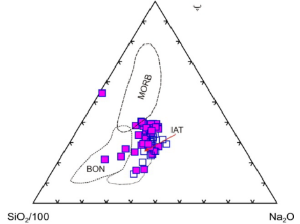
شکل ۱۱ نمودارهای رده‌بندی زمین‌ساختی الف) و ب- برگرفته از [۳۸]، پ و ت برگرفته از مرجع [۳۹] برای کلینوپیکروکسن‌های منطقه مورد بررسی.
