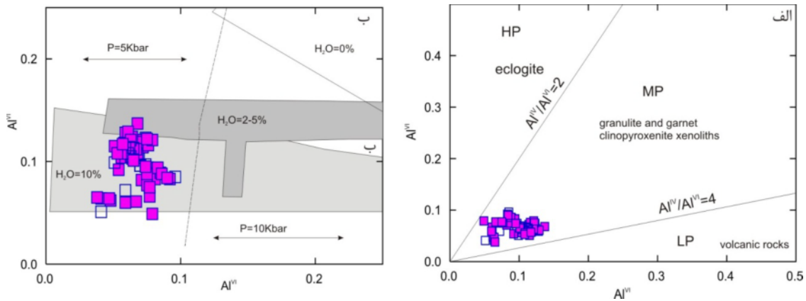
شکل ۹ الف- نمودار تغییرات Al^{VI} نسبت به Al^{IV} برای برآورد فشار تشکیل کلینوپيروکسن [۳۴]. (HP=میدان فشار بالا، MP=میدان فشار متوسط و LP=میدان فشار پایین). ب- نمودار توزیع آلومینیوم در جایگاه چاروچی و هشت وجهی، مقدار آب ماگما هنگام تبلور در حدود ۱۰٪ و فشار محیط تبلور کمتر از ۵ کیلو بار است [۳۷].
