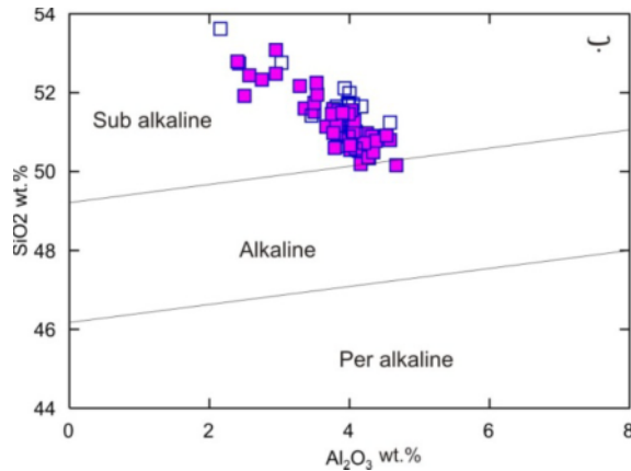
شکل ۱۰ نمودار تفکیک الف) Ti نسبت به Ca+Na [۳۶] و ب) SiO 2 نسبت به Al 2 O 3 [۲۸] برای کلینوپیکروکسن‌های مورد بررسی.
