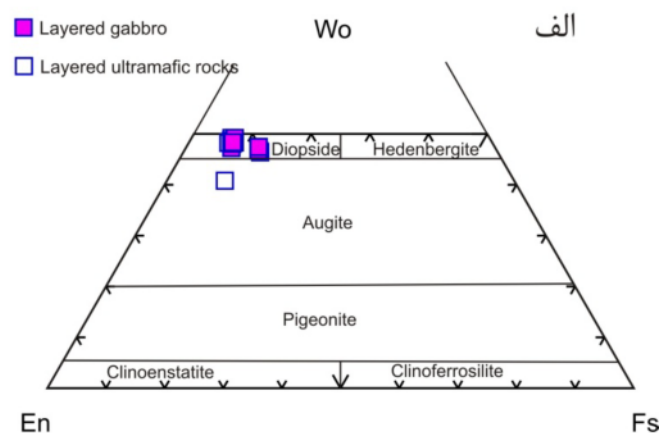
شکل ۴ موقعیت کلینوپیروکسن‌های گابروهای لایه‌ای جنوب ارزوهی الف- در نمودار En-Fs-Wo [۱۶] و ب- در نمودار J-Q [۱۶]. (Q=Ca+Mg+Fe 2+ )
