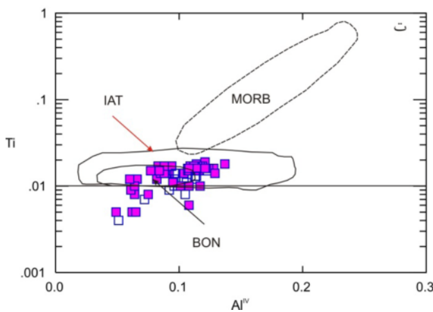
شکل ۱۱ نمودارهای رده‌بندی زمین‌ساختی الف) و ب- برگرفته از [۳۸]، پ و ت برگرفته از مرجع [۳۹] برای کلینوپیکروکسن‌های منطقه مورد بررسی.
