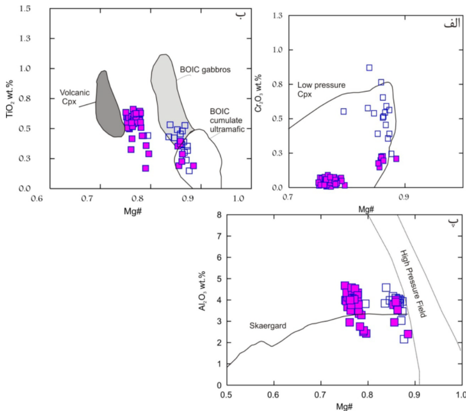
شکل ۷ نمودارهای الف) Cr_2O_3 ، ب) TiO_2 و پ) Al_2O_3 نسبت به Mg\# . گستره‌های مربوط به شکل‌های الف و ب برگرفته از مرجع [۲۰] است. گستره فشارهای بالا برگرفته از [۲۶] و گستره اسکارگارد برگرفته از مرجع [۲۷] است.
