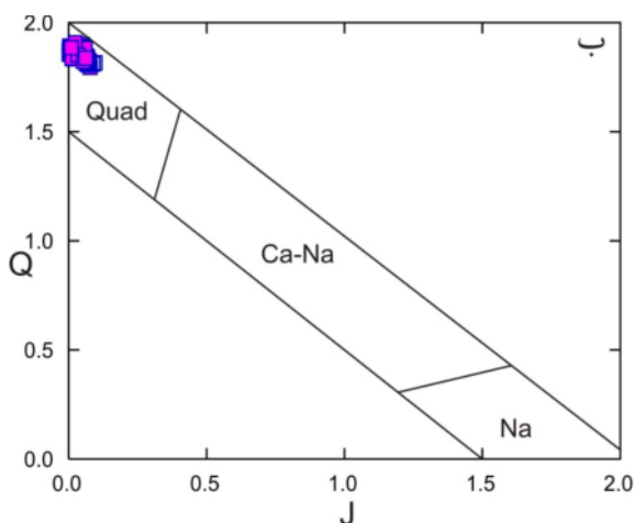
شکل ۴ موقعیت کلینوپیروکسن‌های گابروهای لایه‌ای جنوب ارزوهی الف- در نمودار En-Fs-Wo [۱۶] و ب- در نمودار J-Q [۱۶]. (Q=Ca+Mg+Fe 2+ )
