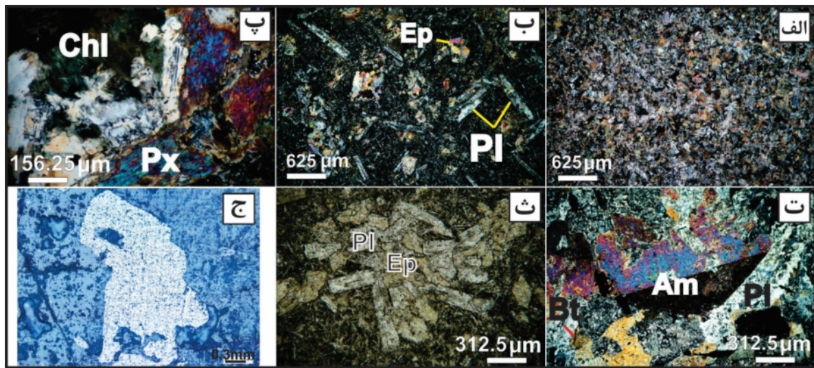
شکل ۳ تصاویر سنگ‌نگاری از سنگ‌های مافیک مورد بررسی. الف- بافت دانهریز (xpl). ب- بافت پورفیری یا بلاستوپورفیری (xpl). پ- پیروکسن‌های نسبتاً سالم که در حال دگرسان شدن هستند در کنار کلریت‌های ثانویه (xpl). ت- آمفیبول‌ها کاملاً شکلدار و احتمالاً اولیه با ماکل دوتایی و در حال تجزیه شدن به همراه آمفیبول هورنبلند و پلاژیوکلاز کاملاً دگرسان شد. مرکز کاملاً به کانی‌های ثانوی از جمله اپیدوت و کانی‌های کدر و کناره به آلبیت تبدیل شده است (xpl). ث- بافت گلوپورپورفیری دربردارنده کانی‌های پلاژیوکلاز اولیه و اپیدوت ثانویه (ppl). ج- کانی‌سازی هماتیت و اکسیدهای آهن به صورت پرشوندگی در اثر دگرسانی (PPL).
