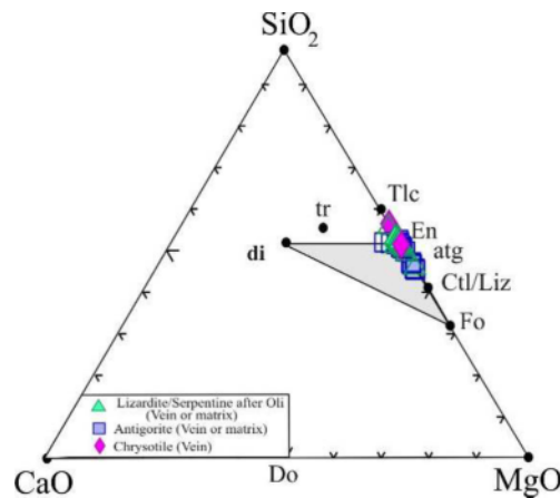
شکل ۱۳ سیستم MgO-SiO 2 -CaO و نتایج تجزیه سرپانتین‌های مجموعه افیولیتی صحنه بر آن.
