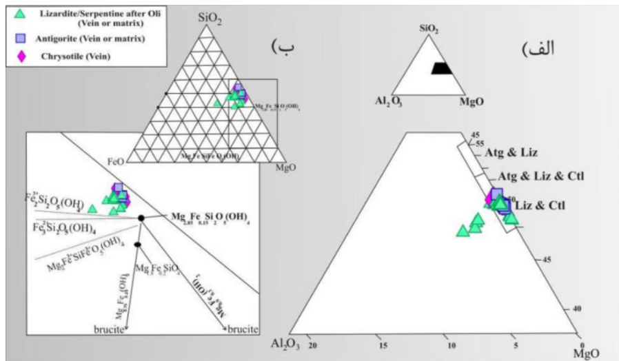
شکل ۱۴ الف- گستره پایداری کانی‌های گروه سرپانتین بر سیستم MgO-SiO 2 -Al 2 O 3 . ب- براساس سیستم سه تایی MgO-SiO 2 -FeO سرپانتین نمونه‌های مورد بررسی بر ضلع MgO-SiO 2 واقع شده‌اند.
