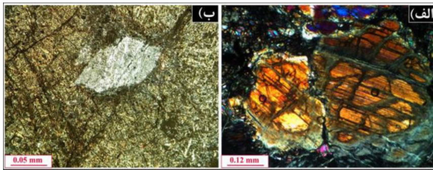
شکل ۷ الف- تشکیل باسیت در راستای شکستگی‌های ارتوپروکسن. ب- جایگزینی ارتوپروکسن توسط آنتی‌گوریت.
