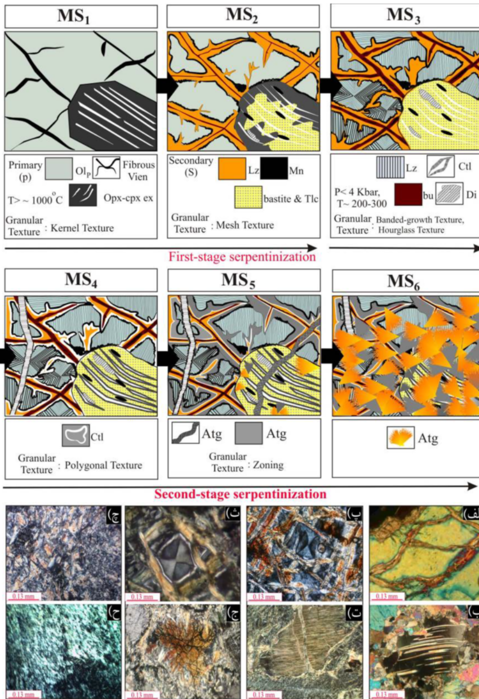
شکل ۹ طرحواره و تصویر واقعی مراحل پیشرفت سرپانتینیته شدن پریدوتیت‌های سرپانتینیته مجموعه افیولیتی صحنه. مرحله ۱- ایجاد شکستگی‌های کرنل در بلورهای الیوین. مرحله ۲- شروع سرپانتینیته شدن و تشکیل لیزاردیت در شکستگی‌های اولیه. الف و ب- تصاویر واقعی مراحل یک و دو که در پریدوتیت‌های سرپانتینیته مجموعه افیولیتی صحنه دیده می‌شود. مرحله ۳- افزایش رشد رگه‌های لیزاردیتی به سمت مرکز بلور الیوین و جایگزینی کامل الیوین و ایجاد بافت‌های نواری، شبکه‌ای و ساعت‌شنی. پ و ت- تصاویر پریدوتیت‌های سرپانتینیته مجموعه افیولیتی صحنه که پیشرفت سرپانتینیته شدن آن‌ها معادل مرحله سه است. مرحله ۴- رشد رگه کریزوتیل بر چند وجهی‌های کاملاً لیزاردیتی شده. رگه‌های کریزوتیل در اطراف بافت شبکه‌ای نیز گسترش یافته‌اند. مرحله ۵- رشد رگه آنتی‌گوریت و گسترش در اطراف بافت شبکه‌ای. ث و ج- تصاویر پریدوتیت‌های سرپانتینیته مجموعه افیولیتی صحنه که نشان‌دهنده مراحل چهار و پنج سرپانتینیته شدن است. مرحله ۶- گسترش آنتی‌گوریت‌های شعله‌ای بر زمینه که با از بین رفتن بافت و کانی‌های اولیه و ثانویه همراه است. چ و ح- تصاویر واقعی مرحله ششم است که در پریدوتیت‌های سرپانتینیته مجموعه افیولیتی صحنه موجود است.
