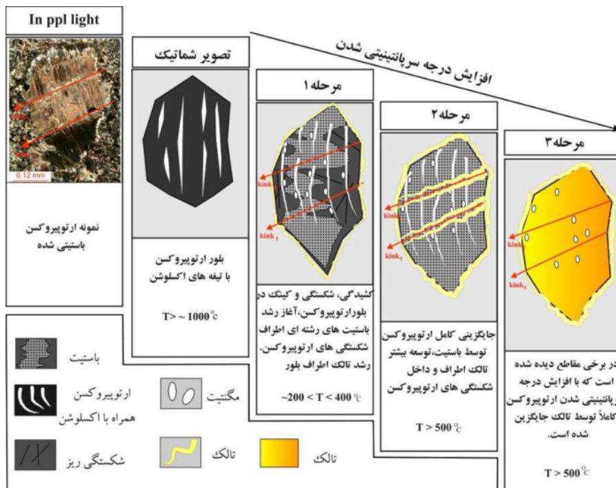
شکل ۸ مراحل دگرسانی ارتوپروکسن در سنگ‌های هارزبورژیتی مجموعه افیولیتی صحنه [۱۴].
