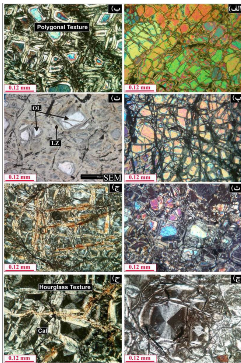
شکل ۶ سازوکار سرپانتینی شدن الیوین. الف، ب، پ- ایجاد شکستگی‌های چند وجهی و رشد لیزاردیت. ت- تصویر SEM از چگونگی تشکیل بافت شبکه‌ای. ث، ج- نمونه‌ای از بافت شبکه‌ای در سنگ‌های گروه دو و سه. چ، ح- بافت ساعت شنی.
