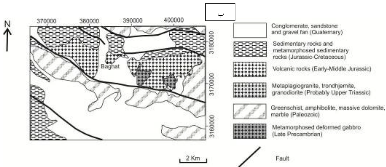
شکل ۱ الف- موقعیت منطقه مورد بررسی بر نقشه ایران، ب- نقشه ساده شده زمین شناسی باغات (۱:۱۰۰۰۰۰) [۸].
