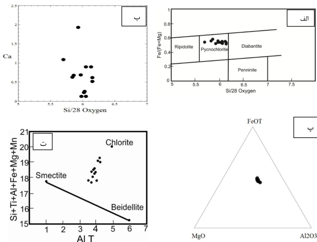
شکل ۴ نمونه‌های مورد بررسی بر الف) نمودار رده‌بندی کلریت‌ها [۱۳] و ب) نمودار Ca-Si، پ- نمونه کلریت‌های مورد بررسی بر نمودار MgO-FeO ۱ -Al ۲ O ۳ (ت) گستره ترکیبی کلریت‌های مورد بررسی [۳۰]، این کلریت‌ها دارای لایه‌هایی از کانی‌های اسمکتیت هستند.
