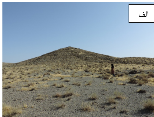
شکل ۲ الف- نمایی از گنبد داسیتی در منطقه باغات، ب- نمایی از برگراری زمین ساختی تکتونیکی در سنگهای داسیتی منطقه باغات.
