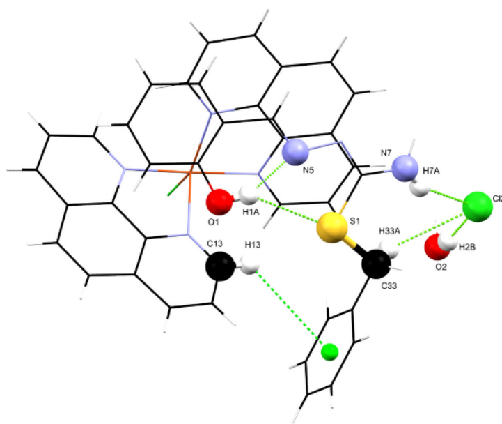
شکل ۲ برهم کنش های درون مولکولی در ترکیب [\text{Cu}(\text{Phen})_2\text{Cl}]\cdot\text{H}_2\text{L}\cdot\text{Cl}\cdot\text{H}_2\text{O} .
