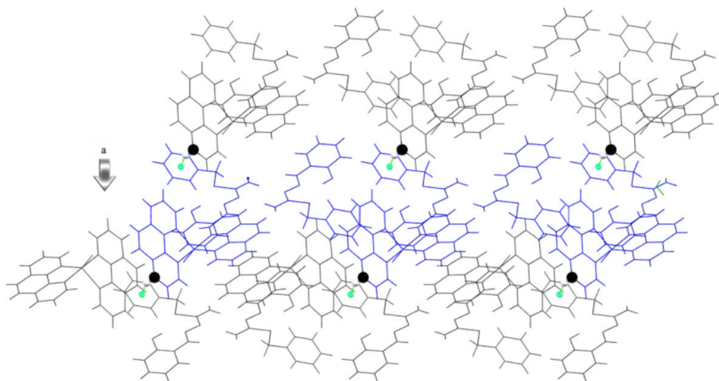
شکل ۴ رشد دو بعدی کمپلکس [\text{Cu}(\text{Phen})_2\text{Cl}]\cdot\text{H}_2\text{L}\cdot\text{Cl}\cdot\text{H}_2\text{O} در راستای a از طریق برهم کنش \text{C20-H20}\cdots\pi: \text{C34-C39}^{\text{iii}} (symmetry code iii: x, y, 1+z ).
