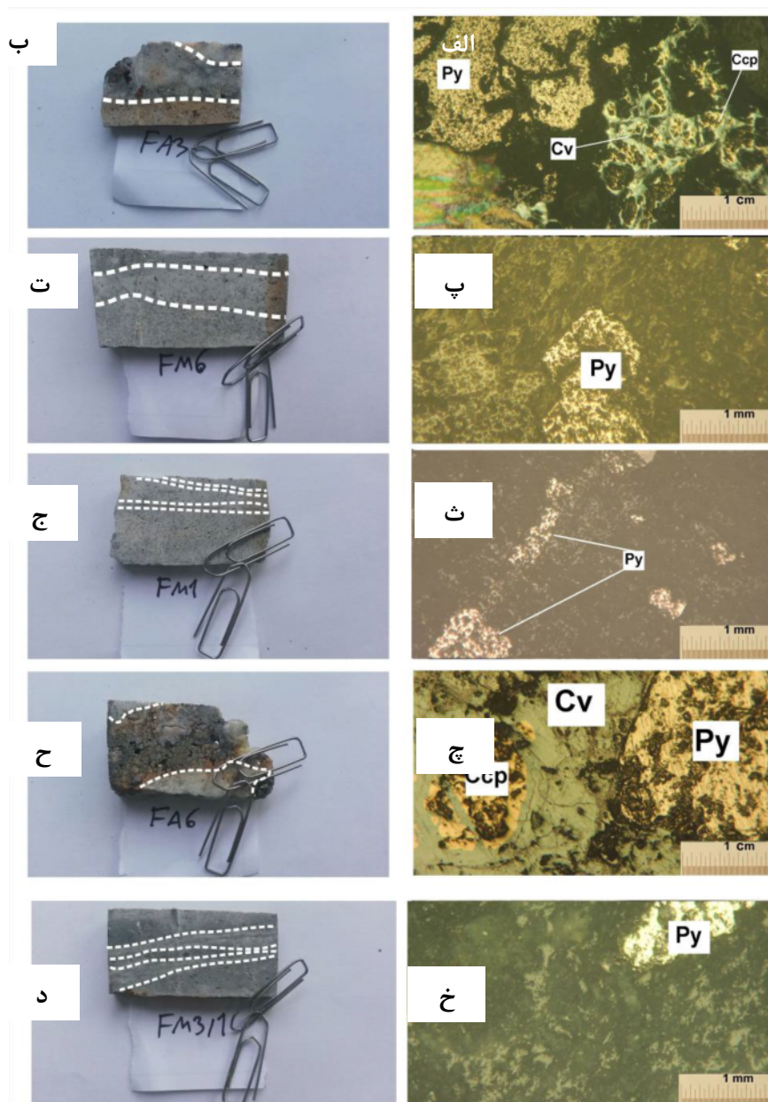
شکل ۶ تصاویر نمونه دستی و مقاطع میکروسکوپی رگچه‌های مختلف در منطقه فیروزه-قیچی. الف) رگچه کوارتز-پیریت-کالکوپیریت-تورمالین در نور بازتابی، ۲۰ تا ۲۵ درصد کالکوپیریت به کاولیت تبدیل شده است. ب) نمونه دستی رگچه نوع I (پ) رگچه کوارتز-کلریت-پیریت-تورمالین در نور بازتابی که پیریت شکلدار کاملاً مشخص است. ت) نمونه دستی رگچه نوع II (ث) رگچه کوارتز-پیریت در نور. ج) نمونه دستی رگچه نوع III (چ) رگچه کوارتز-پیریت-کالکوپیریت در نور بازتابی. کالکوپیریت تا ۸۰ درصد به کاولیت تبدیل شده است. ح) نمونه دستی رگچه نوع IV (خ) رگچه کوارتز-تورمالین-پیریت در نور بازتابی (د) نمونه دستی رگچه نوع V. Py: پیریت، Cv: کاولیت، Ccp: کالکوپیریت. علائم اختصاری برگرفته از مرجع
