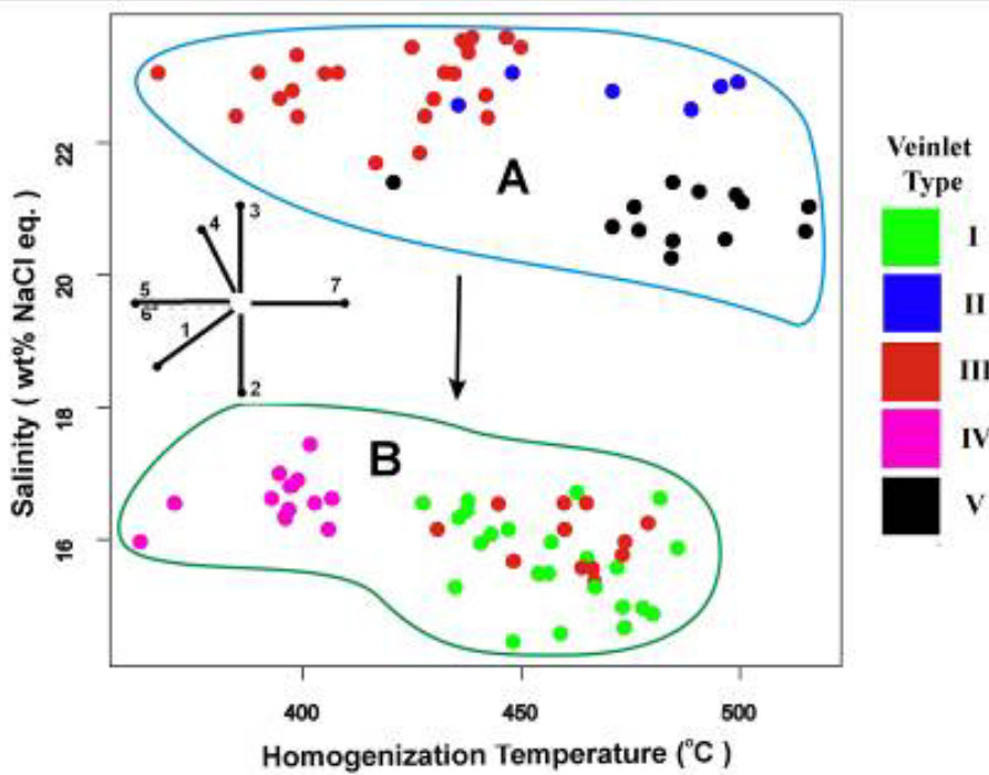
شکل ۹ نمودار شوری نسبت به دمای همگن شدگی انواع سیال‌های درگیر کانسار کوه زر (منطقه فیروزه-قیچی). روندهای ممکن تکامل سیال در نمودار دما-شوری برگرفته از مرجع [۱۷] است. روند ۱- آمیختگی سیال A با سیال سردتر و شوری کمتر B، روندهای ۲ و ۳- آمیختگی سیال A با سیال‌های دیگر با شوری مختلف ولی دمای یکسان. روند ۴- شوری فاز باقی‌مانده در اثر جوشش افزایش پیدا کرده است. روند ۵- سردشدگی سیال. روند ۶- باریک شدگی سیال‌های درگیر و روند ۷- تراوش سیال‌های درگیر طی گرمایش.
