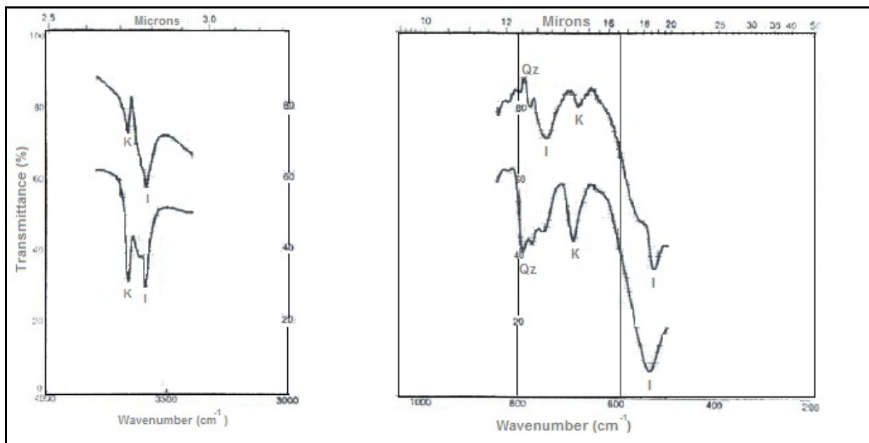
شکل ۳ طیف جذبی ایلیت: I پیش (نوارهای پائینی) و پس (نوارهای بالائی) از حذف کانی‌های همراه کوارتز (Qz) و کائولینیت (K).
