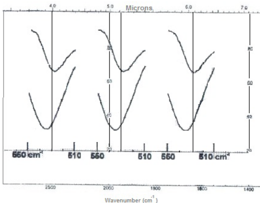
شکل ۴ طیف جذبی ۵ بار بزرگ شده ایلیت در گستره 550-510 \text{ cm}^{-1} (ارتعاش \text{Al}^{\text{VI}}\text{-O-Si} ) پیش (نوارهای پائینی) و پس (نوارهای بالائی) از حذف کانی‌های همراه.
