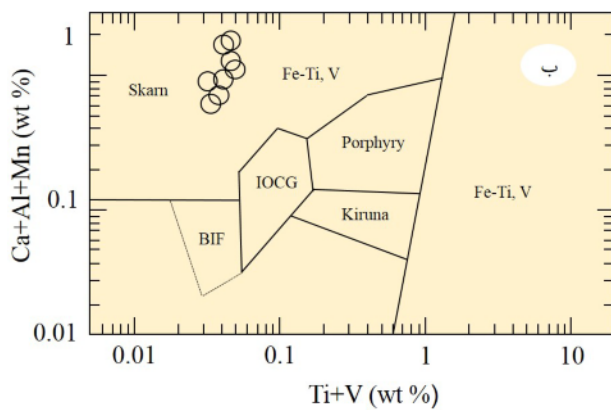
شکل ۱۰ الف) نمودار تغییرات Ti+V نسبت به Ni/(Cr+Mn) که نشان دهنده ارتباط نمونه‌های کانسار آهن دردروی با کانسار نوع اسکارن است، ب) نمودار تغییرات Ti+V نسبت به Ca+Al+Mn که قرار گرفتن کانسار دردروی در گستره‌ی اسکارن را نشان داده است [۲۴].
