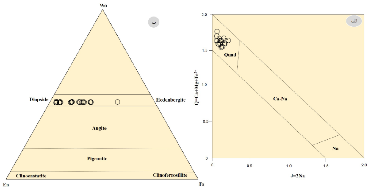
شکل ۷ الف) نمودار J-Q [۲۱] که نشان می‌دهد که کلینوپیروکسن‌های اسکارن دردوی در گستره‌ی پیروکسن‌های Ca-Fe-Mg قرار می‌گیرند و ب) کلینوپیروکسن در کانسار اسکارن دردوی از نوع دیوپسید و هدنبرژیت بوده که در گستره‌ی کانسارهای اسکارن آهن متداول است.
