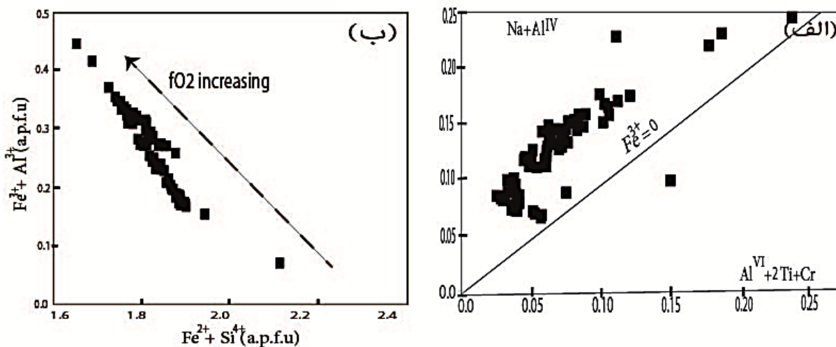
شکل ۶ نمودار Na+Al IV نسبت به Al VI +2Ti+Cr برای تعیین گریزندگی اکسیژن در محیط تشکیل کلبیوپروکسن که شرایط اکسیدی در محیط تبلور این کانی‌ها را نشان می‌دهد [۱۹] و ب) نمودار Fe 2+ +Si 4+ نسبت به Fe 3+ [۲۳].
