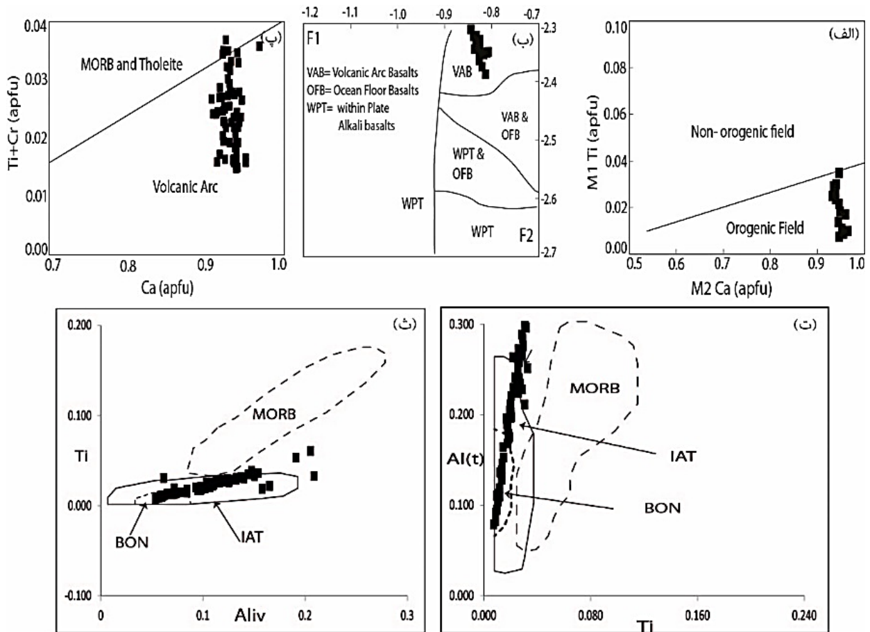
شکل ۵ ترکیب کلبیوپروکسن‌های موجود در سنگ‌های بازالتی پیرانشهر جهت تعیین محیط زمین ساختی. الف) نمودار Ti نسبت به Ca [۱۴]، ب) نمودار F1 نسبت به F2 [۱۵]، پ) نمودار Ti+Cr نسبت به Ca [۱۴]، ت و ث) نمودارهای تعیین محیط زمین ساختی بر اساس ترکیب کانی کلبیوپروکسن [۱۶]، IAT: تولیت جزایر قوسی، BON: بونینیت، MORB: بازالت پشته میان اقیانوسی.
