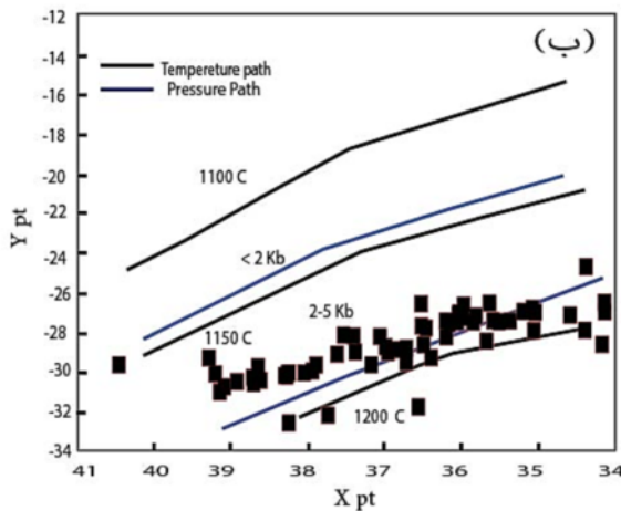
شکل ۷ الف) نمودار توزیع آلومینیوم در جایگاه چهاروجهی و هشت وجهی [۲۴] و ب) نمودار تعیین دما و فشار براساس ترکیب کلاینوپيروكسن [۲۵].
