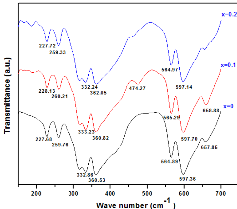
شکل ۳ طیف‌های تبدیل فوریه فروسرخ دور نمونه‌های \text{Sb}_x\text{Y}_{3-x}\text{Fe}_5\text{O}_{12} با مقادیر جانمایی (۰/۲، ۰/۱، ۰) (x).
