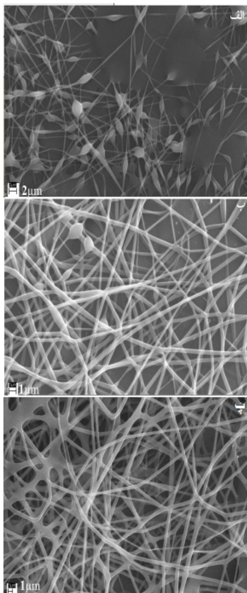
شکل ۵ تصویر SEM الیاف الکتروپرسی شده با پلیمر PVA با غلظت الف (۵٪ وزنی ب) ۷٪ وزنی و پ (۷/۵ درصد وزنی).
