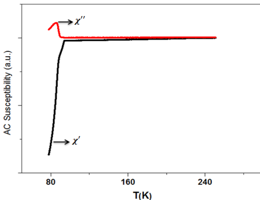
شکل ۱۵ منحنی پذیرفتاری مغناطیسی ac الیاف ابرسانا.
