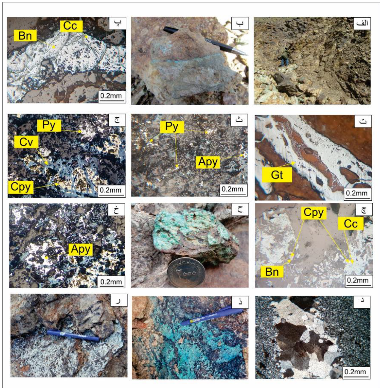
شکل ۴ کانی‌سازی منطقه زاوه. الف) رخنمون رگه کانی‌سازی. ب) بافت رگچه‌ای کریزوکلا. پ) بافت رگچه‌ای بورنیت و کالکوزیت. ت) رگچه گوتیت. ث) پیریت و آرسنوپیریت با بافت پراکنده. ج) بافت جانشینی کوولیت و بافت توده‌ای پیریت. چ) بافت جانشینی کالکوزیت و بورنیت. ح) بافت گل کلمی مالاکیت. خ) آرسنوپیریت با بافت توده‌ای و پراکنده. د) رگچه سیلیس. ذ) رخنمون صحرایی آزوریت. ر) نمایی از کات کبود. مالاکیت = Mlc، آرسنوپیریت = Apy، پیریت = Py، کالکوپیریت = Cpy، کالکوزیت = Cc، بورنیت = Bn، کوولیت = Cv و گوتیت = Gt. [۱۳].
