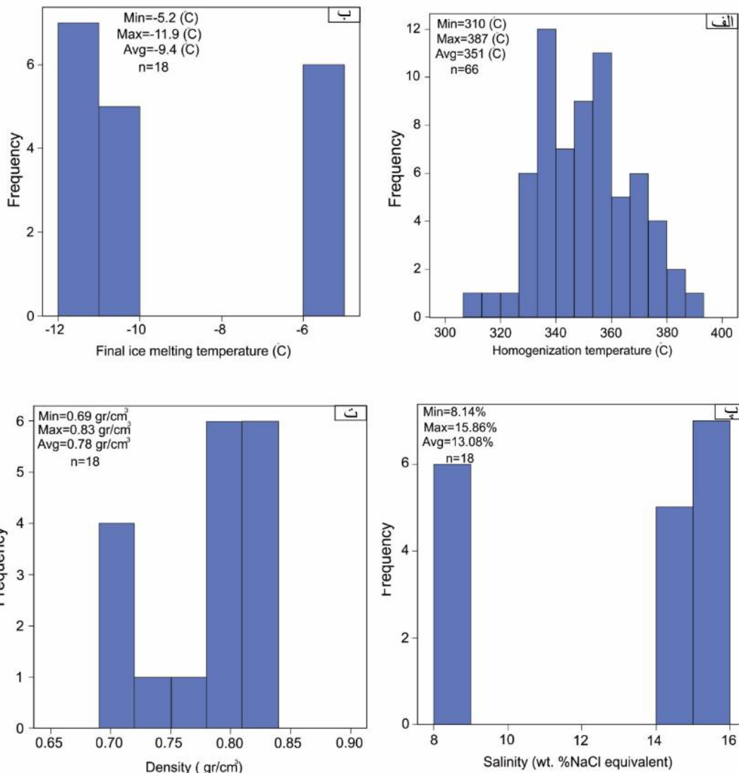
شکل ۷ نمودارهای ستونی مربوط به تجزیه سیال‌های درگیر منطقه زاوه. الف) نمودار ستونی دمای همگن‌شدگی. ب) نمودار ستونی آخرین دمای ذوب یخ. پ) نمودار ستونی مقدار شوری. ت) نمودار ستونی مقدار چگالی.
