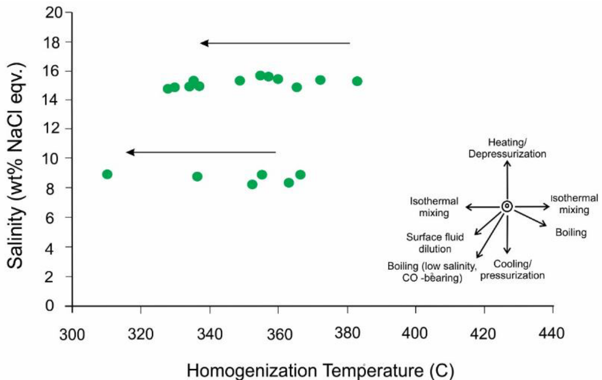
شکل ۹ نمودار شوری-دما همگن‌شدگی سیال‌های درگیر منطقه زاوه. روندهای ممکن تکامل سیال در نمودار دما-شوری برگرفته از مرجع [۱۵].
