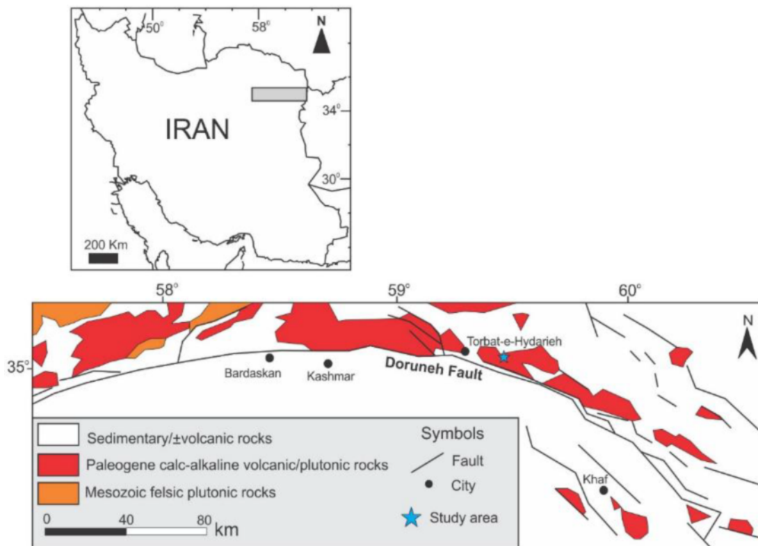
شکل ۱ موقعیت کمر بند ماگمایی خواف-کاشمر- بردسکن در شمال شرقی ایران و نقشه زمین شناسی ساده شده آن همراه با موقعیت منطقه زاوه
