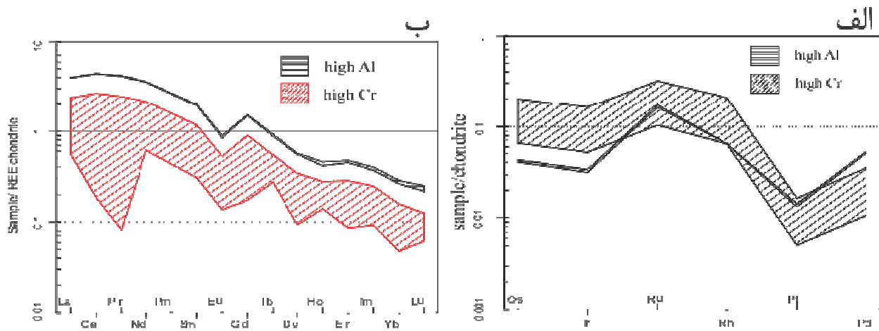
شکل ۳ الف) الگوی الگوی PGE و الف) REE بهنجار شده نسبت به کندریت [۱۵] برای کرومیت‌های سبزوار. تفاوت دو گروه کرومیت‌های غنی از آلومینیوم و غنی از کروم کاملاً نمایان است.
