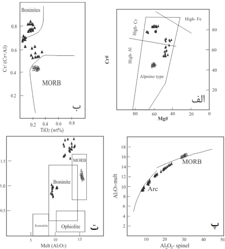
شکل ۶ نمودارهای تفکیک نوع ماگمای اولیه برای کرومیت‌های سبزوار بر اساس ترکیب بلورهای کرومیت. الف) نمودار Mg# نسبت به Cr# (۱۷۸). ب) نمودار TiO 2 نسبت به Cr# (۱۷). پ) نمودار Al 2 O 3 محاسبه شده برای مذاب نسبت به Al 2 O 3 کرومیت (۱۹). ت) نمودار اکسید آلومینیوم نسبت به FeO/MgO محاسبه شده برای مذاب [۱۷]. علائم همانند شکل ۴ است.
