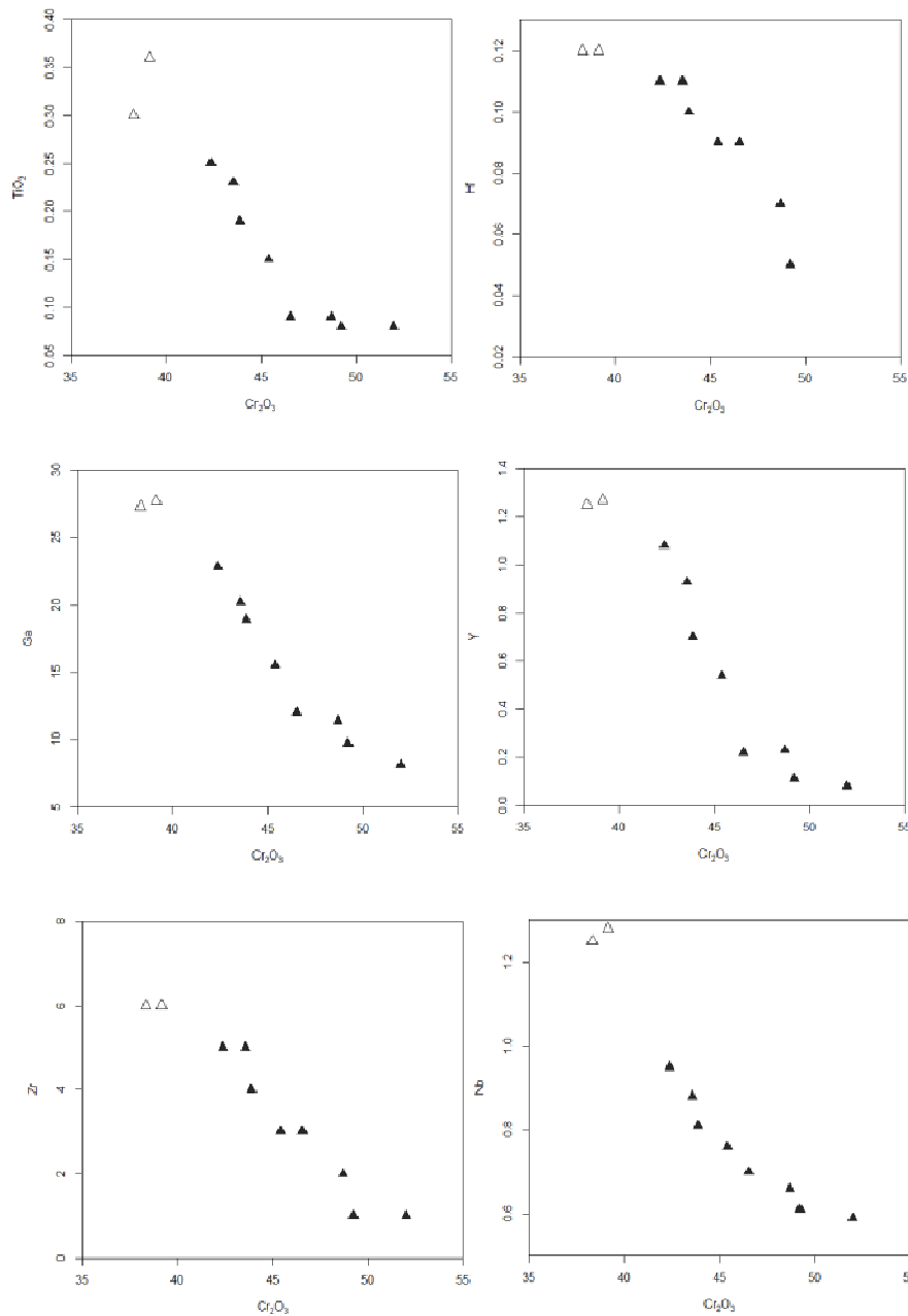
شکل ۵ نمودارهای دوتایی Cr 2 O 3 در برابر عناصر کمیاب برای کرومیت‌های سبزوار. علائم به کار رفته مانند شکل ۴ است.
