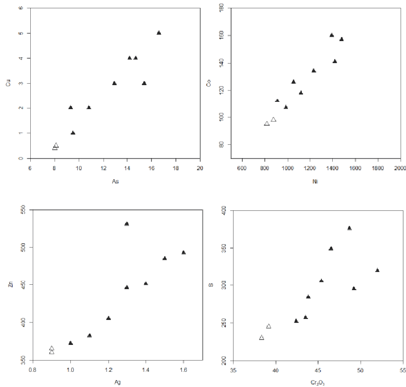
شکل ۴ نمودارهای دوتایی تفکیک ترکیب کرومیت‌های غنی از آلومینیوم ( \Delta ) و غنی از کروم ( \blacktriangle ) در کرومیت‌های سبزوار. غلظت Cr_2O_3 به درصد وزنی و سایر عناصر به ppm است.
