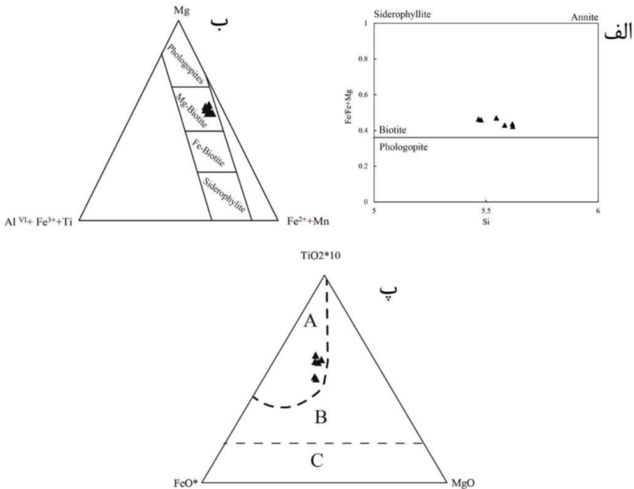
شکل ۳ رده بندی میکاهای باتولیت ممزار براساس ترکیب شیمیایی آن‌ها (الف) با استفاده از نمودار مرجع [۵] و (ب) - [۵]؛ (پ) - رده بندی انواع بیوتیت‌ها به سه گروه بیوتیت‌های اولیه (A)؛ بیوتیت‌های ثانویه (B)؛ بیوتیت‌های باز تبلور یافته (C) [۶].
