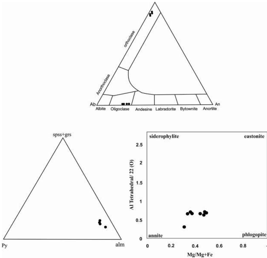
شکل ۵ ترکیب شیمیایی کانی‌ها در میگماتیت‌های بروجرد: الف) ترکیب شیمیایی پلاژیوکلازها و فلدسپارهای قلیایی در نمودارهای سه تایی Or, Ab, An [۲۶]، ب) ترکیب شیمیایی گارنت نمودار سه تایی Fe, Mg, Mn+Ca [۲۷] و پ) ترکیب شیمیایی بیوتیت‌ها در نمودار Mg/Mg+Fe نسبت به Al Tetrahedral/22(O) چاروچی که بین قطب فلوگوپیت و آنیت قرار گرفته‌اند
