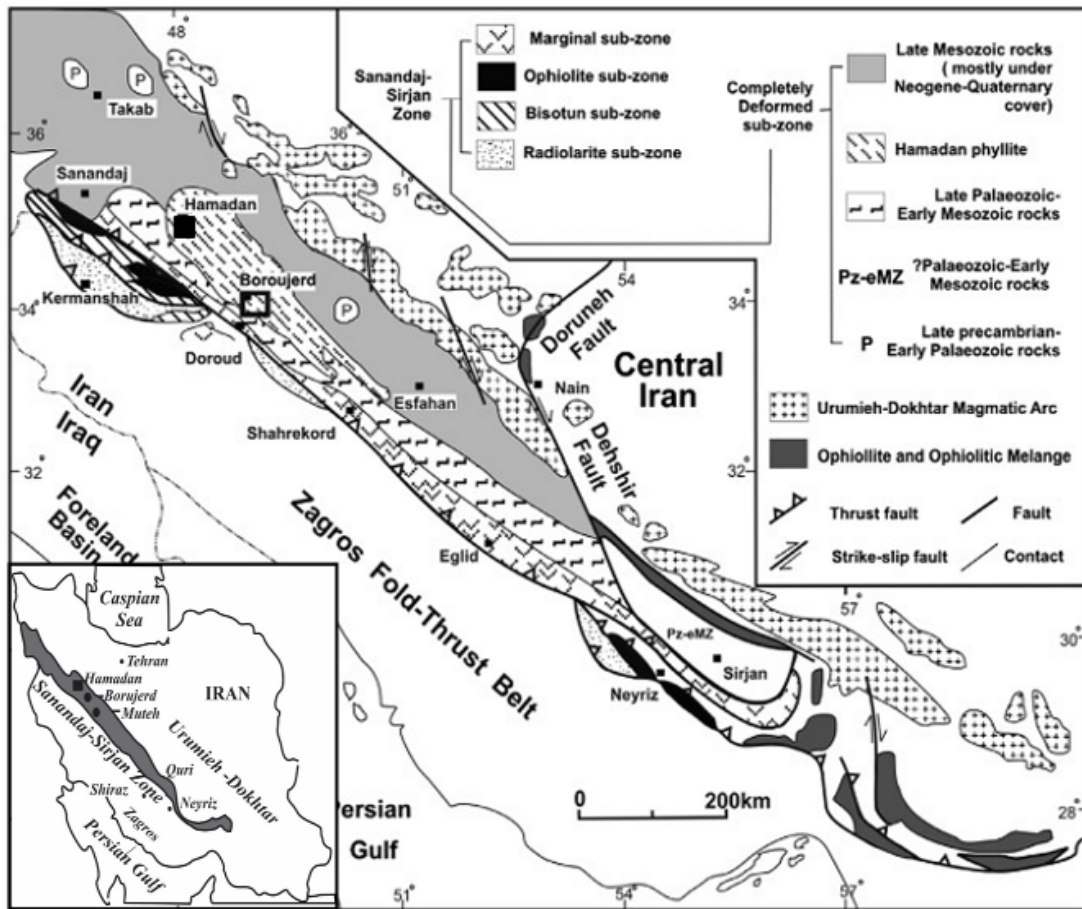
شکل ۱ جایگاه منطقه مورد بررسی در نقشه زمین‌شناسی ایران و جایگاه زمین‌ساختی پهنه‌ها در غرب ایران [۱۴].
