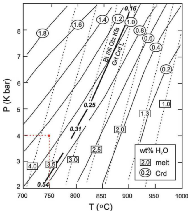
شکل ۹ نمودار تعیین مقدار آب موجود در مذاب و مقدار آب موجود در کزدیریت‌ها با استفاده از مدل ارائه شده در مراجع [۳۶، ۲۹].
