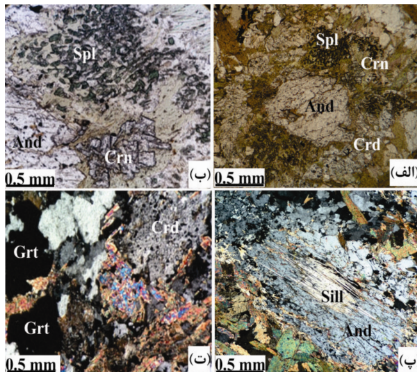
شکل ۴ تصاویر میکروسکوپی از میگماتیت‌های منطقه: الف و ب) سنگ‌های دارای هم رشدی کوردیریت و اسپینل و کروندم اطراف آندالوزیت (در نور ppl)، پ) تبدیل آندالوزیت به سیلیمانیت (در نور xpl) و ت) سنگ‌های دارای کوردیریت همراه با گارنت (در نور xpl).
