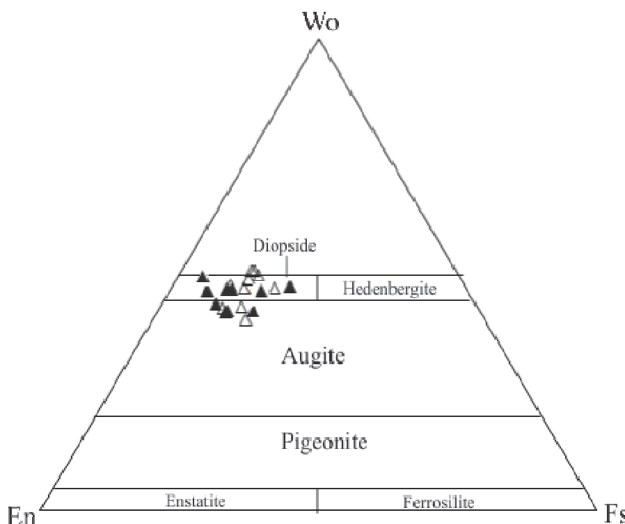
شکل ۳ نمایش ترکیب کلیئوپیروکسن‌های گابروهای پیرانشهر در نمودار رده بندی پیروکسن‌ها [۱۷]. ▲ = کلیئوپیروکسن‌ها در گابروهای قلیایی؛ △ = کلیئوپیروکسن‌ها در گابروهای آهکی قلیایی.
