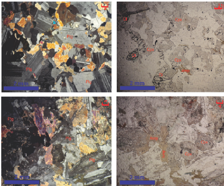
شکل ۲ تصاویری از بافت میکروسکوپی گابروهای پسته: الف و ب) گابروی قلیایی به ترتیب در نور PPL نور XPL؛ پ و ت) گابروی آهکی قلیایی به ترتیب در نور PPL و نور XPL. (Cpx = کلینوپيروكسن؛ Amp = آمفیبول؛ Ol = الیون؛ Plg = پلاژیوکلاز).
