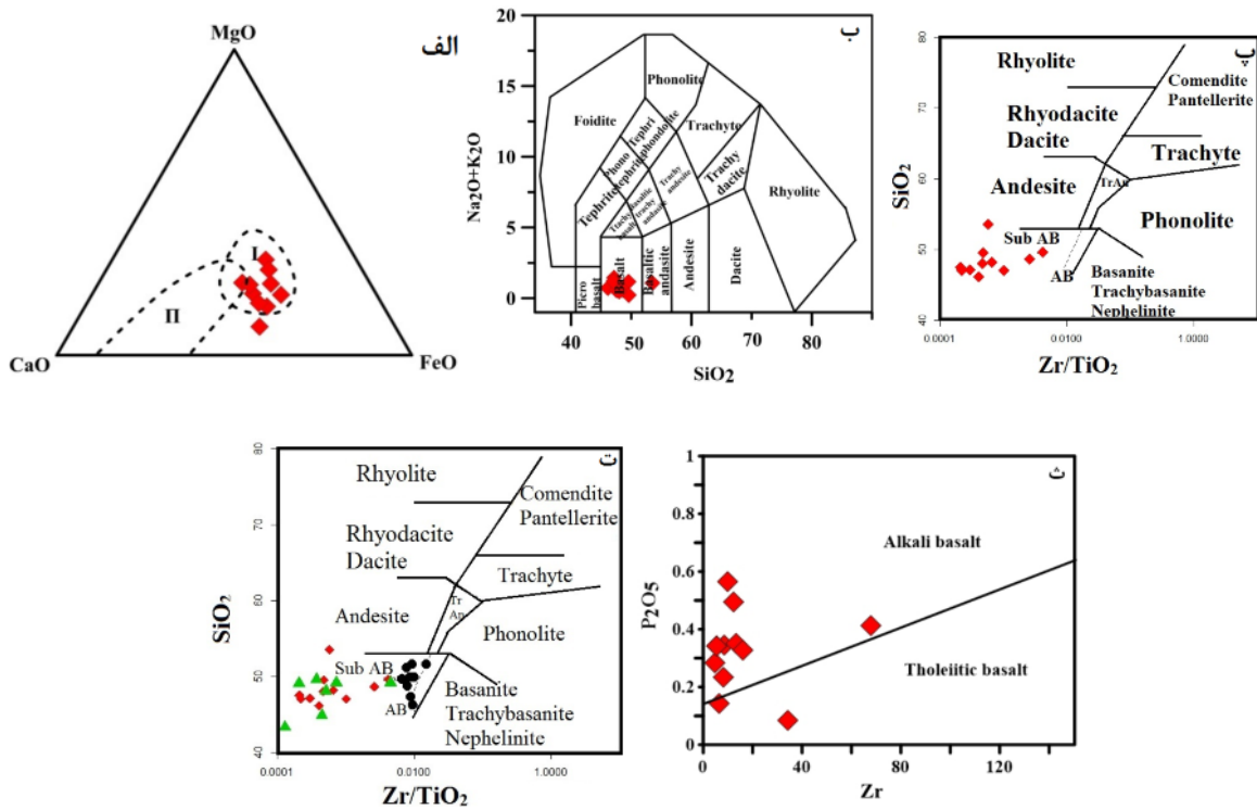
شکل ۴ جایگاه نمونه‌های متابازیتی مجموعه دگرگونی ماجراد در: الف- نمودار مثلثی مرجع [۲۱] جهت تفکیک ارتوآمفیبولیت‌ها (I) و پارآمفیبولیت‌ها (II)، ب - نمودار Na_2O+K_2O نسبت به SiO_2 [۲۲]، پ) نمودار SiO_2 نسبت به Zr/TiO_2 [۲۳] به منظور نامگذاری سنگ‌های آذرین بیرونی مادر متابازیت‌ها، ت) نمودار مرجع [۲۳] جهت مقایسه موقعیت ترکیبی متابازیت‌های ماجراد و شترکوه، (دایره‌های سیاه رنگ) و جندق (مثلث‌های سبز رنگ) و ث) نمودار P_2O_5 نسبت به Zr برای تعیین سری ماگمایی [۲۳].
