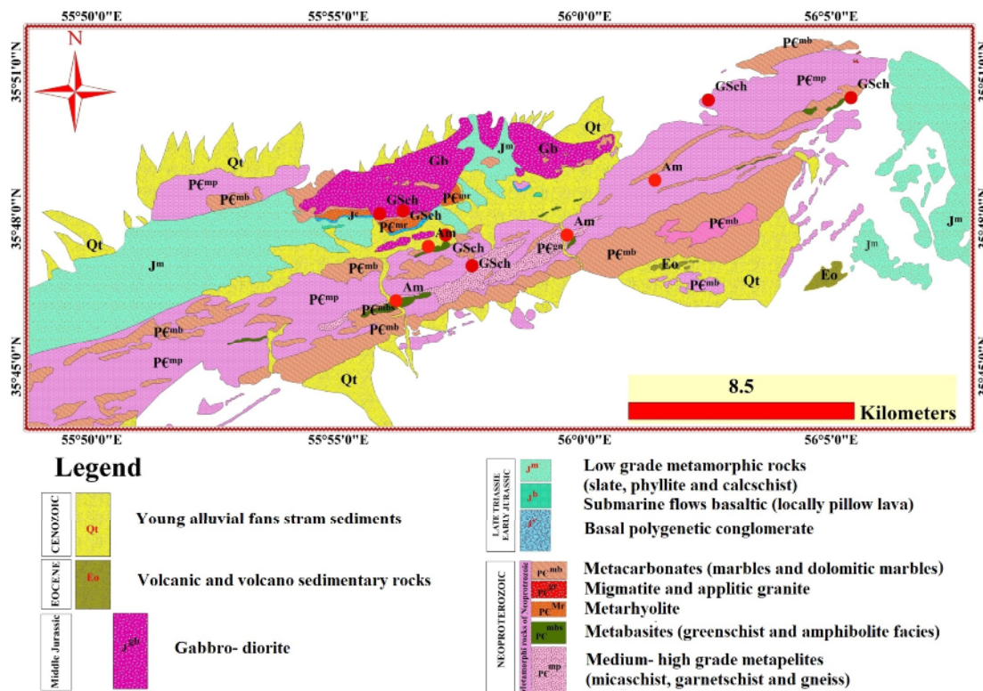
شکل ۱ نقشه زمین‌شناسی مجموعه دگرگونی ماجراد بر پایه برداشت‌های صحرائی، تصاویر ماهواره‌ای گوگل ارث و نتایج سن‌سنجی ایزوتوپی جدید که موقعیت جغرافیایی و ترکیب سنگ‌شناسی نمونه‌های متابازیتی مورد بررسی بر آن مشخص شده است (دایره‌های قرمز رنگ با علامت اختصاری GSch نشانگر شیبست سبز و Am نشانگر آمفیبولیت هستند).
