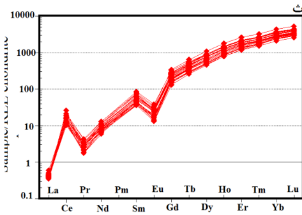
شکل ۷ الف- تصاویر کاتدولومینسانس زیرکن های جدا شده از نمونه متابازیتی (آمفیبولیت) مجموعه دگرگونی ماجراد که سن های به دست آمده برای هر نقطه از زیرکن ها بر آنها مشخص شده است. ب و پ) نمودار سازگاری و میانگین سنی رسم شده بر اساس نتایج تجزیه های ایزوتوپی به روش LA-ICPMS. ت) نمودار ستونی نشان دهنده تغییرات سنی زیرکن های استخراج شده از متابازیت های ماجراد و ث) نمودار تغییرات عناصر خاکی نادر بهنجار شده نسبت به کندریت [۲۴] برای زیرکن های استخراج شده از نمونه آمفیبولیتی تعیین سن شده.
