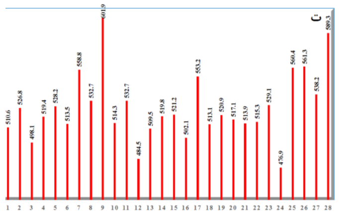
شکل ۷ الف- تصاویر کاتدولومینسانس زیرکن های جدا شده از نمونه متابازیتی (آمفیبولیت) مجموعه دگرگونی ماجراد که سن های به دست آمده برای هر نقطه از زیرکن ها بر آنها مشخص شده است. ب و پ) نمودار سازگاری و میانگین سنی رسم شده بر اساس نتایج تجزیه های ایزوتوپی به روش LA-ICPMS. ت) نمودار ستونی نشان دهنده تغییرات سنی زیرکن های استخراج شده از متابازیت های ماجراد و ث) نمودار تغییرات عناصر خاکی نادر بهنجار شده نسبت به کندریت [۲۴] برای زیرکن های استخراج شده از نمونه آمفیبولیتی تعیین سن شده.
