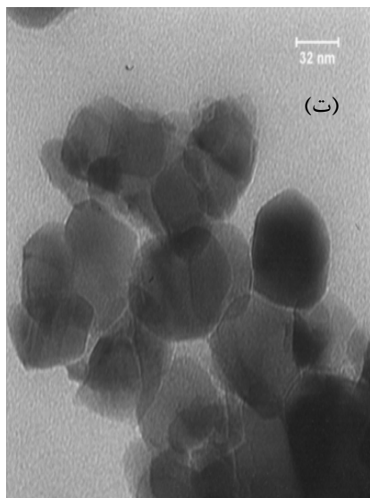
شکل ۳ تصاویر TEM نمونه‌های \text{TiO}_2 با ۱٪ کروم بازیخت شده در الف) 400^\circ\text{C} و ب) 800^\circ\text{C} و با ۵٪ کروم در دمای بازیخت (پ) 400^\circ\text{C} و ت) 800^\circ\text{C}
