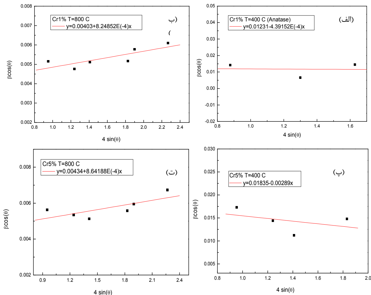
شکل ۲ نمودارهای برازش شده به روش ویلیامسون-هال برای نمونه‌های TiO_2 (الف) ۱٪ کروم در دمای ۴۰۰ °C، (ب) ۱٪ کروم در دمای ۸۰۰ °C، (پ) ۵٪ کروم در دمای ۴۰۰ °C، (ت) ۵٪ کروم در دمای ۸۰۰ °C.
