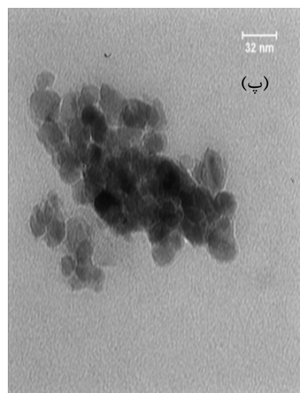
شکل ۳ تصاویر TEM نمونه‌های \text{TiO}_2 با ۱٪ کروم بازیخت شده در الف) 400^\circ\text{C} و ب) 800^\circ\text{C} و با ۵٪ کروم در دمای بازیخت (پ) 400^\circ\text{C} و ت) 800^\circ\text{C}
