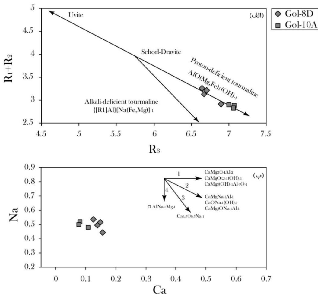
شکل ۶ الف) جانشینی کاتیون‌های مورد بررسی با استفاده از نمودارهای R_1+R_2 نسبت به R_3 ( R_1=Ca+Na ، R_2=Fe+Mg+Mn ) و (ب) بررسی جانشینی کاتیون با استفاده از نمودار Na نسبت به Ca (برگرفته از مرجع [۳۷]).
