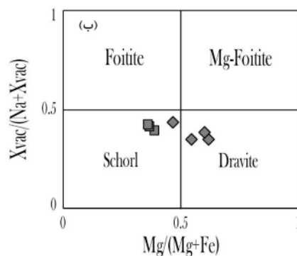
شکل ۴ الف) نمودار \text{Na}/(\text{Na}+\text{Ca}) نسبت به \text{Fe}/(\text{Fe}+\text{Mg}) (برگرفته از مرجع [۳۵]) و ب) نمودار X\text{-vacancy}/(\text{Na}+X\text{-vacancy}) نسبت به \text{Mg}/(\text{Mg}+\text{Fe}) (برگرفته از مرجع [۹]).
