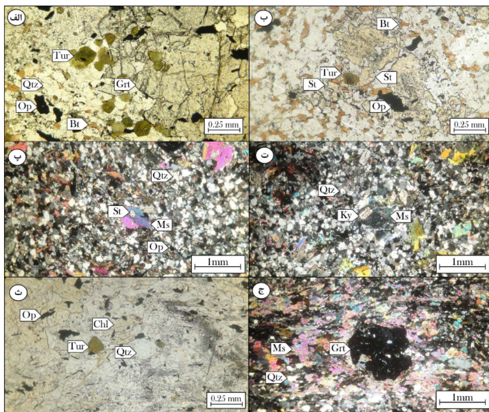
شکل ۲ الف) تورمالین‌های شکل‌دار و نیمه‌شکل درون گارنت و در زمینه سنگ (نور PPL)، ب) تورمالین درون استارولیت (نور PPL)، پ) استارولیت درون مسکوویت (نور XPL)، ت) کیانیت در مسکوویت (نور XPL)، ث) تورمالین‌های نیمه‌شکل تا بی‌شکل در زمینه سنگ (نور PPL)، ج) گارنت شکل‌دار (نور XPL) علائم اختصاری کانی‌ها به جز Op (کانی‌های تیره) از مرجع [۳۲] گرفته شده است.
