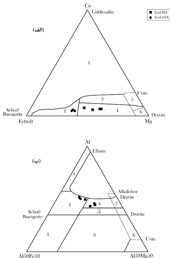
شکل ۵ شیمی تورمالین در سنگ‌های مختلف (الف) و ب) ۱: گرانیوتوئیدها، پگماتیت‌ها و آپلیت‌های غنی از لیتیم، ۲: گرانیوتوئیدهای فقیر از لیتیم و پگماتیت‌ها و آپلیت‌های وابسته، ۳: سنگ‌های کوارتز-تورمالین‌دار غنی از آهن، ۴: متاپلیت‌ها و متاسمیت‌های در تعادل با یک فاز سیال غنی از آلومینیوم، ۵: متاپلیت‌ها و متاسمیت‌های در تعادل با یک فاز سیال فقیر از آلومینیوم، ۶: سنگ‌های آهکی سیلیکاته، ۷: سنگ‌های دگر-فرامافیک با کلسیم پائین و دگررسوب‌های غنی از وانادیم و کروم و ۸: کربناتیت‌ها و پیروکسنیت‌های دگرگون‌شده (برگرفته از مرجع [۳۵]).
