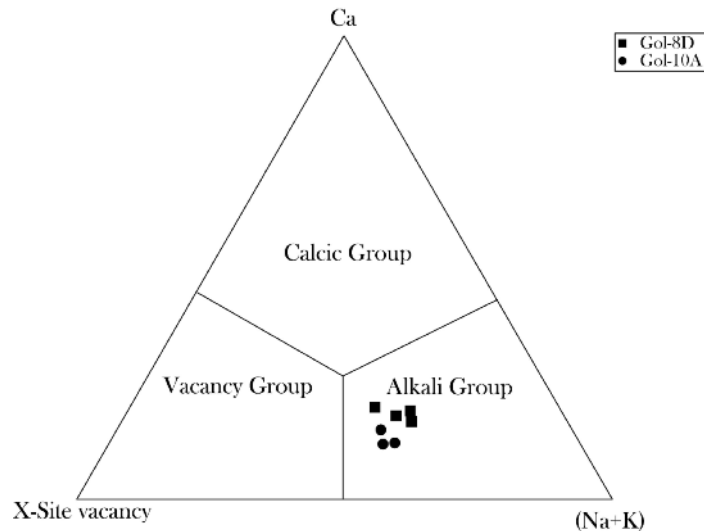
شکل ۳ رده‌بندی تورمالین‌ها بر اساس نمودار \text{Ca}-(\text{Na}+\text{K}) تهیجای جایگاه X (برگرفته از مرجع [۹]).
