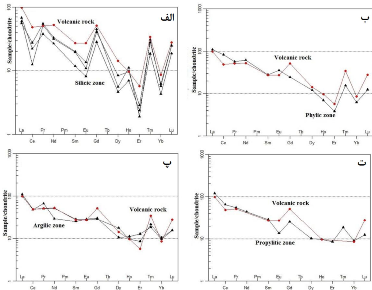
شکل ۴ مقایسه الگوی پراکندگی عناصر خاکی نادر بهنجار شده به کدریت در سنگ‌های آتشفشانی منطقه، (الف) نمونه‌های پهنه سیلیسی، (ب) پهنه فیلیک، (پ) پهنه آرژیلی، (ت) پهنه پروپیلیتی.
