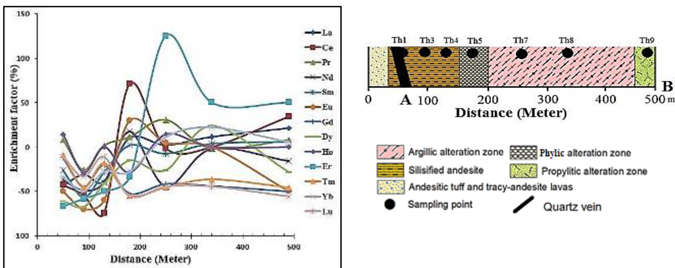
شکل ۵ نمودارهای توزیع عناصر خاکی نادر در پهنه‌های دگرسانی از سمت سنگ‌های دیواره به سمت پهنه‌های دگرسانی.
