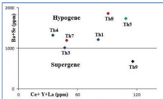
شکل ۷ نمودار (Ce+Y+La) - (Ba+Sr) [۳۳] جهت تعیین نوع محلول‌های دگرسان‌کننده در منطقه زایلک.
