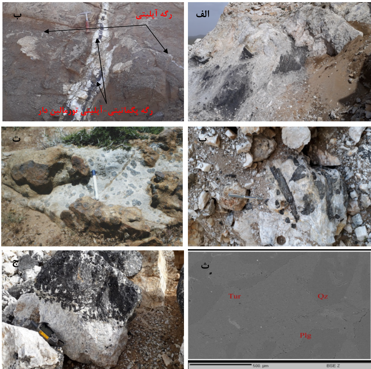
شکل ۲ الف) تصویر صحرایی پگماتیت‌های دربردارنده تورمالین و مسکوویت‌های بسیار دانه درشت (دید به سمت شرق)، ب) تصویر صحرایی رگه‌های آپلیتی و آپلیتی-پگماتیته تورمالین‌دار که در سنگ‌های گرانودیوریتی برونزد دارند (دید به سمت غرب)، پ) تصویر صحرایی پگماتیت‌های دربردارنده تورمالین و مسکوویت‌های بسیار دانه درشت با روند شمال غربی- جنوب شرقی که پیرامون توده ملاطاب به خوبی دیده می‌شوند. این تورمالین‌ها خود شکل و به صورت تیغه‌های منفرد هستند (دید به سمت جنوب)، ت) تصویر صحرایی تورمالین‌های گرهمی همراه با کوارتز و فلدسپات در گرانیت‌ها (دید به سمت جنوب غرب)، ث) تصویر ریزپردازش الکترونی از تورمالین به همراه کوارتز و پلاژیوکلاز ج) تصویر صحرایی فلدسپات و تورمالین در دو فاز کاملاً مجزا در کنار یکدیگر (دید به سمت جنوب).
