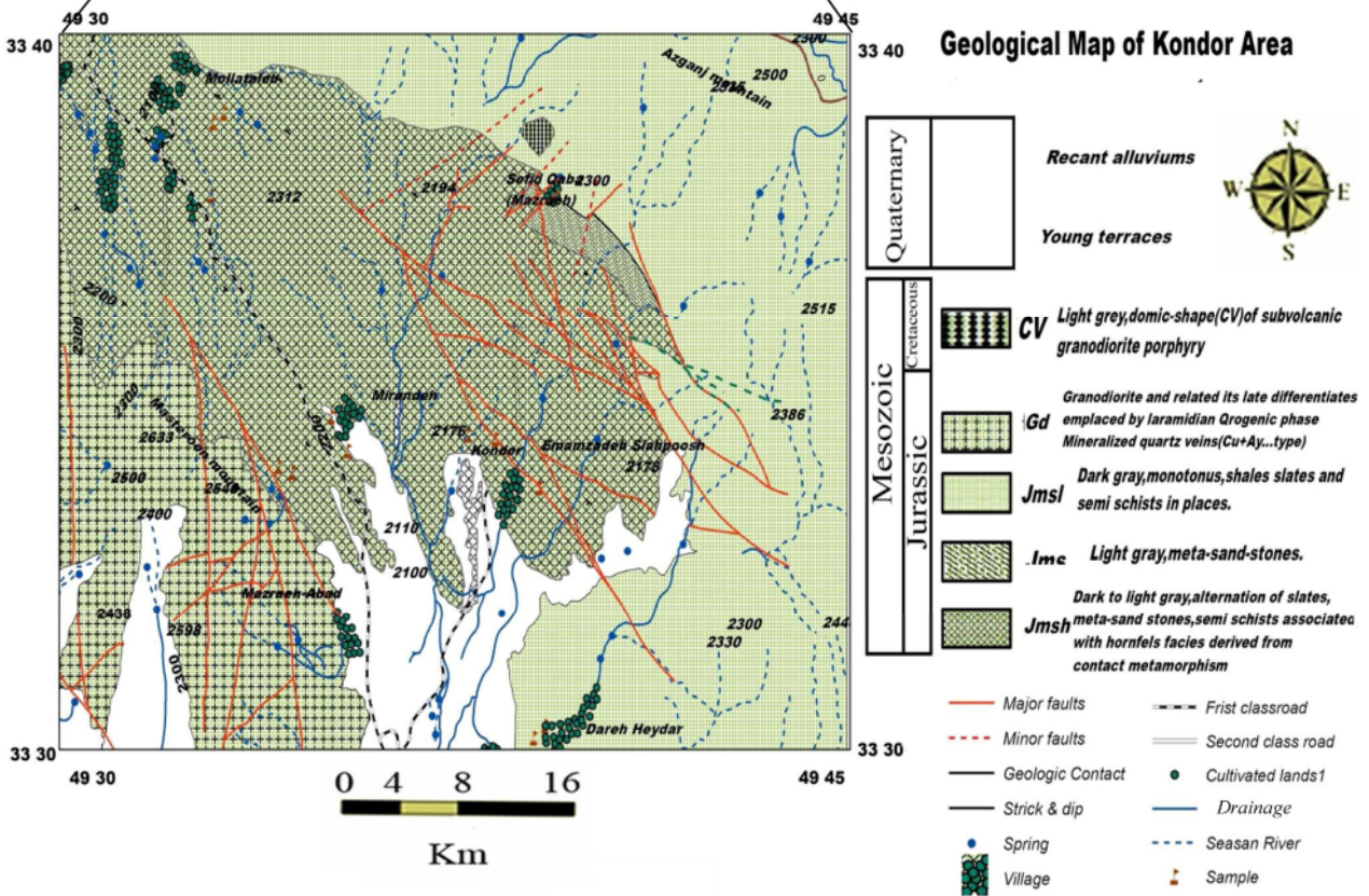
شکل ۱ نقشه زمین‌شناسی ناحیه کندر برگرفته از مرجع [۲۵] با تغییر و جایگاه ناحیه مورد بررسی بر آن
