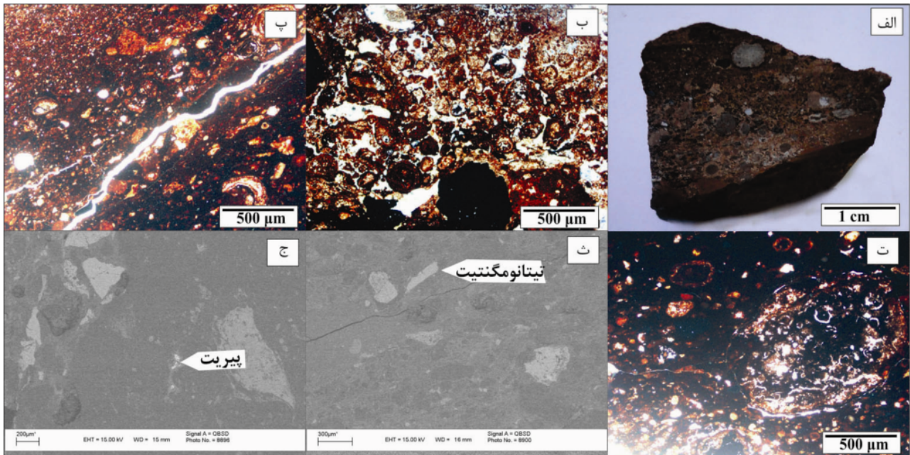
شکل ۴ (الف) تصویر ماکروسکوپی از نمونه کانسنگی شامل قطعات تخریبی گرد شده و پیروییدی در کانسنگ BRO، تصویر میکروسکوپی از (در نور عبوری قطبیده) بافت اویدی-پیروییدی، (ب) بافت ریزدانه ای و رگچه ای، (ت) بافت پلتی در زمینه‌ای ریزدانه ای و اویدی. (ث و ج) تصاویر میکروسکوپی الکترونی روبشی از قطعات تیتانومگنتیت و پیریت.
