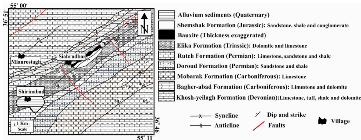
شکل ۲ نقشه زمین‌شناسی نهشته بوکسیتی سیاهرودبار [۱].
