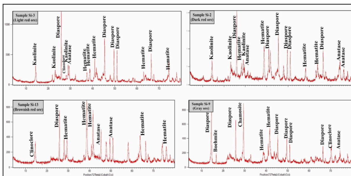
شکل ۵ طیف‌های XRD مربوط به کانسنگ‌های سیاه‌رودبار.
