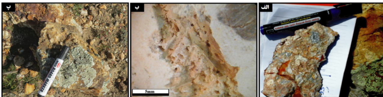
شکل ۱۰ برخی شواهد نشان دهنده جوشش سیال در منطقه: الف) برش گرمایی، ب) کلسیت تیغه‌ای و پ) کوارتز با بافت گل کلمی.
