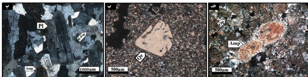
شکل ۲ تصاویر میکروسکوپی از واحدهای سنگی منطقه: الف) کانی آمفیبول در آندزیت، ب) کوارتز خلیجی در ریولیت، پ) بافت دانه‌ای و کانی‌های پلاژیوکلاز و فلدسپار قلیایی در سنگ‌های نفوذی منطقه (Op: کانی‌های کدر، Amp: آمفیبول، Qz: کوارتز، Pl: پلاژیوکلاز، K-Fsp: پتاسیم فلدسپار [۱۲])
