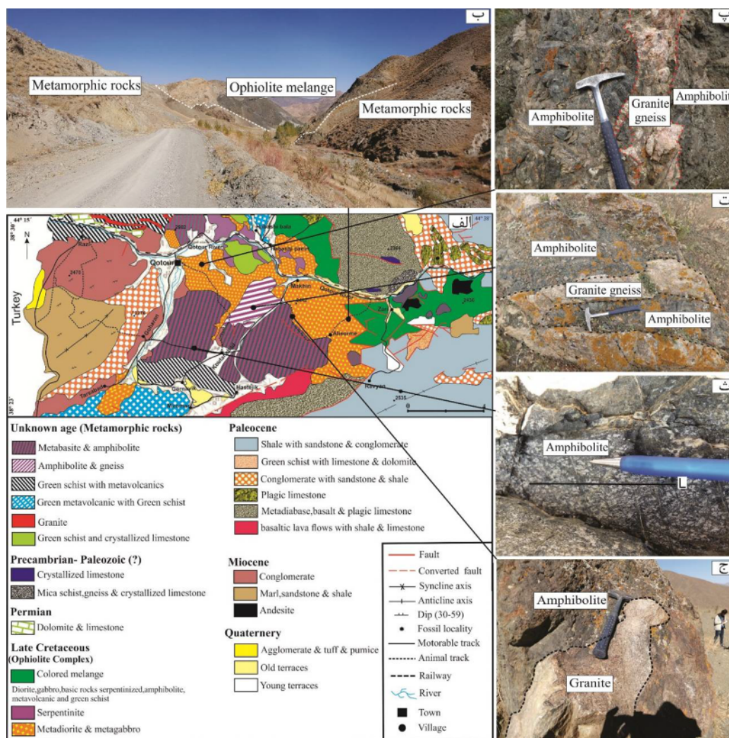
شکل ۱ الف- نقشه زمین‌شناسی منطقه مورد بررسی (برگرفته از نقشه‌های ۱:۱۰۰۰۰۰ خوی و قطور با تغییرات از). ب- مرز بین آمیزه افیولیتی با سن کرتاسه‌ی پسین و سنگ‌های دگرگونی با سن نامشخص مورد بررسی در مسیر روستای علی‌سرمه به زری، (دید به سمت شمال‌شرق)، پ و ت- رخنمون آمفیبولیت با رگه‌های گرانیت‌گنیس در شرق روستای قطور (دید به سمت شمال‌شرق) و شمال‌شرق کوتان‌آباد (دید به سمت شرق). ث- جهت‌یافتگی در آمفیبولیت‌ها و ج- قطعات گرانیتی موجود در آمفیبولیت‌ها در مسیر کوتان‌آباد به علی‌سرمه.
