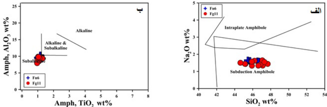
شکل ۵ جایگاه آمفیبول‌های موجود در سنگ‌های دیوریتی کرتاسه پسین جنوب غرب سبزواری (الف) نمودار \text{Na}_2\text{O} نسبت به \text{SiO}_2 [۲۸] و (ب) نمودار ارزیابی ماهیت ماگمای سازنده این سنگ‌ها با استفاده از ترکیب شیمیایی آمفیبول [۲۹].
