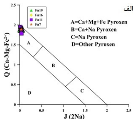
شکل ۶ جایگاه کلینوپیروکسن‌های سنگ‌های دیوریتی کرتاسه پسین جنوب غرب سبزوار در الف) نمودار J-Q [۳۰] و ب) نمودار مثلثی Wo-En-Fs [۳۰].
