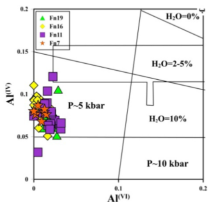
شکل ۱۱ جایگاه کلینوپیروکسن‌های موجود در سنگ‌های دیوریتی کرتاسه پسین جنوب غرب سبزوار در الف) نمودار \text{Al}^{\text{VI}} نسبت به \text{Al}^{\text{IV}} [۴۱] و ب) نمودار \text{Al}^{\text{VI}} نسبت به \text{Al}^{\text{IV}} برای تعیین مقادیر فشار و آب ماگما [۲۸].
