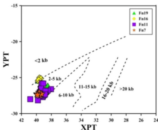
شکل ۱۲ جایگاه کلینوپیروکسن‌های موجود در سنگ‌های دیوریتی کرتاسه پسین جنوب غرب سبزوار در نمودار XPT نسبت به YPT [۴۳].
