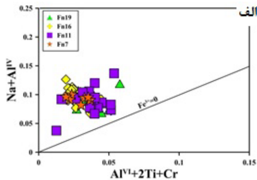
شکل ۷ جایگاه کلینوپیروکسن‌های سنگ‌های دیوریتی کرتاسه پسین جنوب غرب سبزوار در الف) نمودار تعیین‌گریندگی اکسیژن در محیط تبلور پیروکسن‌ها [۳۱] و ب) نمودار تعیین‌میزان اشیاعی در جایگاه چاروچی کلینوپیروکسن‌ها [۳۱].
