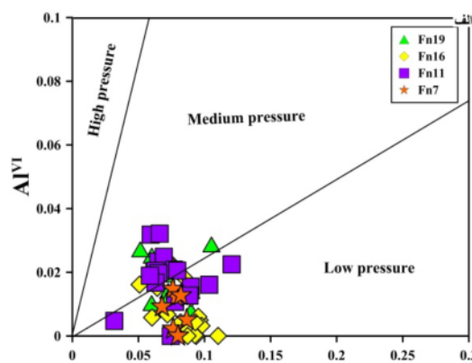
شکل ۱۱ جایگاه کلینوپیروکسن‌های موجود در سنگ‌های دیوریتی کرتاسه پسین جنوب غرب سبزوار در الف) نمودار \text{Al}^{\text{VI}} نسبت به \text{Al}^{\text{IV}} [۴۱] و ب) نمودار \text{Al}^{\text{VI}} نسبت به \text{Al}^{\text{IV}} برای تعیین مقادیر فشار و آب ماگما [۲۸].
