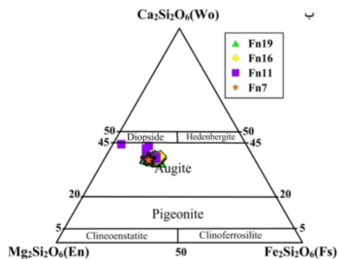
شکل ۶ جایگاه کلینوپیروکسن‌های سنگ‌های دیوریتی کرتاسه پسین جنوب غرب سبزوار در الف) نمودار J-Q [۳۰] و ب) نمودار مثلثی Wo-En-Fs [۳۰].
