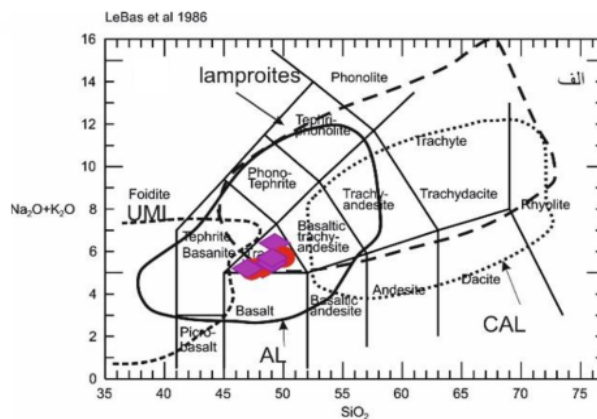
شکل ۳ الف- تقسیم بندی نمونه‌های مورد بررسی در نمودار مرجع [۱۴]. گستره‌های لامپروفیر و لامپروئیت و خط تفکیکی سری‌های ماگمایی برگرفته از مرجع [۱۵] است. (گستره با خطوط پررنگ: ترکیب لامپروفیر قلیایی، گستره با خط چین بزرگ: لامپروفیرهای فرامافیک (UML)، گستره با خط چین ریز: لامپروفیر آهکی قلیایی (CAL) و گستره با نقطه چین: لامپروئیت) ب) نمودار Na_2O+K_2O نسبت به SiO_2 [۱۶]. لامپروفیرها: ● دیابازها: ◆
