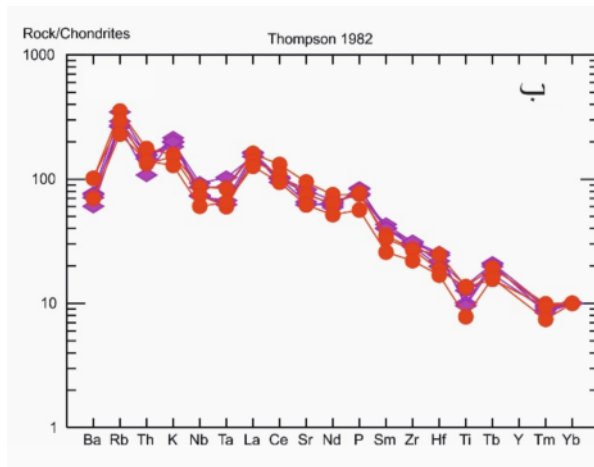
شکل ۴ الف) الگوی REE در سنگ‌های بازالتی قطعه جوپار [۱۷] و ب) نمودار بهنجار شده‌ی سنگ‌های منطقه مورد بررسی نسبت به کندریت [۱۲] علائم مانند شکل ۳ هستند.
