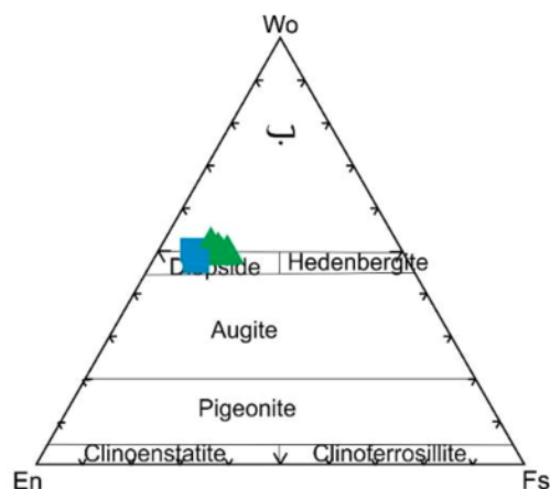
شکل ۵ رده‌بندی پیروکسن‌های منطقه جوپار: الف) ترکیب کلینوپیروکسن‌ها در نمودار Q نسبت به J [۱۸] و ب) نمودار En-Fs- WO [۱۹]. (نمونه‌های دایک دیابازی: ▲. نشانه نمونه‌های دایک لامپروفیری: ■)
