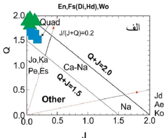
شکل ۵ رده‌بندی پیروکسن‌های منطقه جوپار: الف) ترکیب کلینوپیروکسن‌ها در نمودار Q نسبت به J [۱۸] و ب) نمودار En-Fs- WO [۱۹]. (نمونه‌های دایک دیابازی: ▲. نشانه نمونه‌های دایک لامپروفیری: ■)
