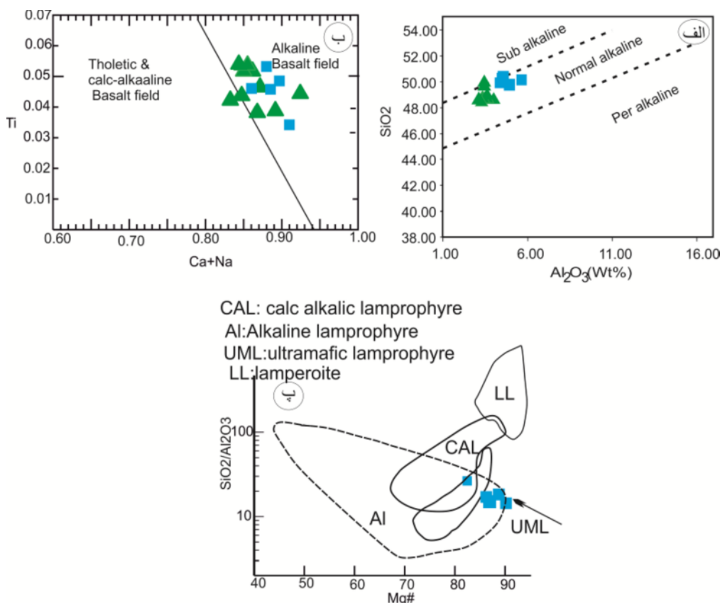
شکل ۶ تعیین سری ماگمایی و جایگاه زمین‌ساختی نمونه‌ها با استفاده از ترکیب شیمیایی پیروکسن در الف) نمودار SiO 2 نسبت به Al 2 O 3 [۲۰]، ب) نمودار Ca+Na در مقابل Ti [۵] و پ) نمودار شناسایی سری ماگمایی لامپروفیرها [۲۴].
