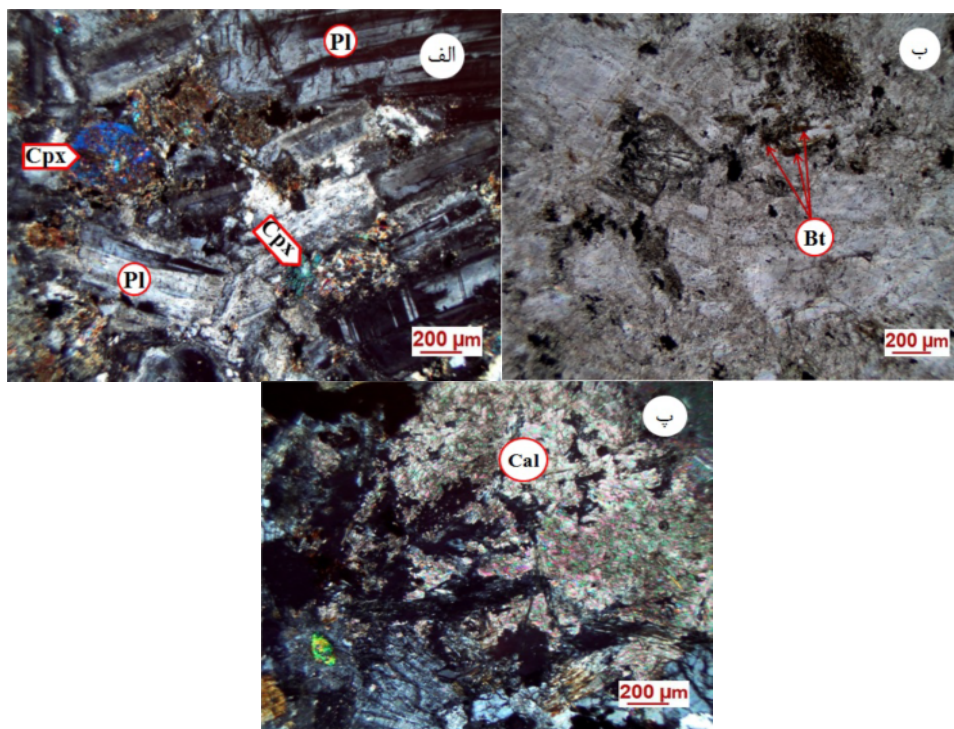
شکل ۲ تصاویر میکروسکوپی سنگ میزبان رگه‌های کوارتز الف) نمایی از بافت دانه‌ای در کوارتز مونزودیوریت، پیروکسن (Cpx) با لبه‌های نیمه گرد شده و بلورهای درشت پلاژیوکلاز رسی شده در نور قطبیده متقاطع (XPL)، ب) کانی بیوتیت (Bt) ثانویه بصورت پراکنده در نور قطبیده صفحه‌ای (PPL) و پ) تشکیل کانی کلسیت (Cal) در بخش‌هایی از سنگ میزبان در نور XPL. علائم اختصاری کانی‌ها برگرفته از مرجع [۲۴] است.
