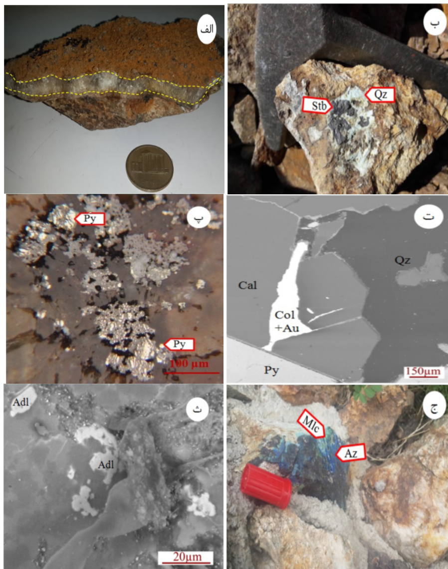
شکل ۴ الف) نمونه دستی از رگه شفاف کوارتز دربردارنده میانبارهای سیال، ب) نمونه دستی کوارتز به همراه کانی استیبینیت (Stb)، ت) تصویر پیریت (Py) در مقطع صیقلی، پ) تصویر میکروسکوپ الکترونی روبشی (SEM) از کانی کلرادوئیت (Col) به همراه طلای آزاد، کوارتز (Qz)، کلسیت (Cal) و پیریت (ث) کانی آدولاریا (Adl) در رگه سیلیسی و ج) نمایی از آثار سطحی کانه‌زایی مس، مالاکیت (Mlc) و آزوریت (Az).
