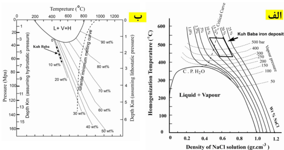
شکل ۱۰ (الف) نمودار دما-چگالی با اعمال شوری برای تعیین مقدار فشار سیال که بین ۳۶۰ تا بیش از ۵۰۰ بار است [۲۵] و (ب) نمودار فشار نسبت به دمای همگن شدگی میانبرهای سیال برای محاسبه عمق کانی سازی [۲۶] (مایع = L، گاز = V، نمک طعام = H، 1Mpa = 10 bars). خطوط پربندی ممتد درصد وزنی نمک طعام حل شده پایدار در بخش مایع سیال درگیر را نشان می دهند.
