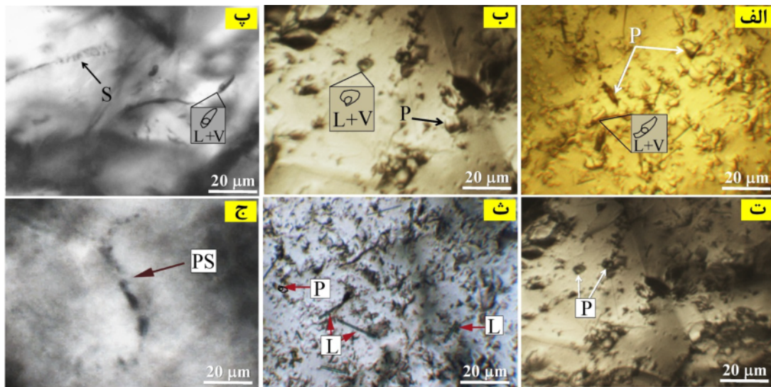
شکل ۷ انواع میانبارهای سیال دیده شده در کانی کوارتز کانسار آهن کوه‌بابا: (الف) میانبارهای سیال اولیه دو فاز (L+V) و تک فاز (S) (ب) میانبارهای سیال دو فاز (L+V)، (پ) میانبارهای سیال دو فاز و میانبارهای سیال ثانویه که در نمونه‌های مورد بررسی بسیار دیده می‌شوند، (ت) میانبارهای سیال دو فاز کوچکتر از ۵ میکرون، (ث) میانبارهای سیال تک فاز (L) که به شکل میله‌ای دیده می‌شوند؛ (ج) میانبار سیال ثانویه کاذب که به شکل S مانند دیده می‌شود.
