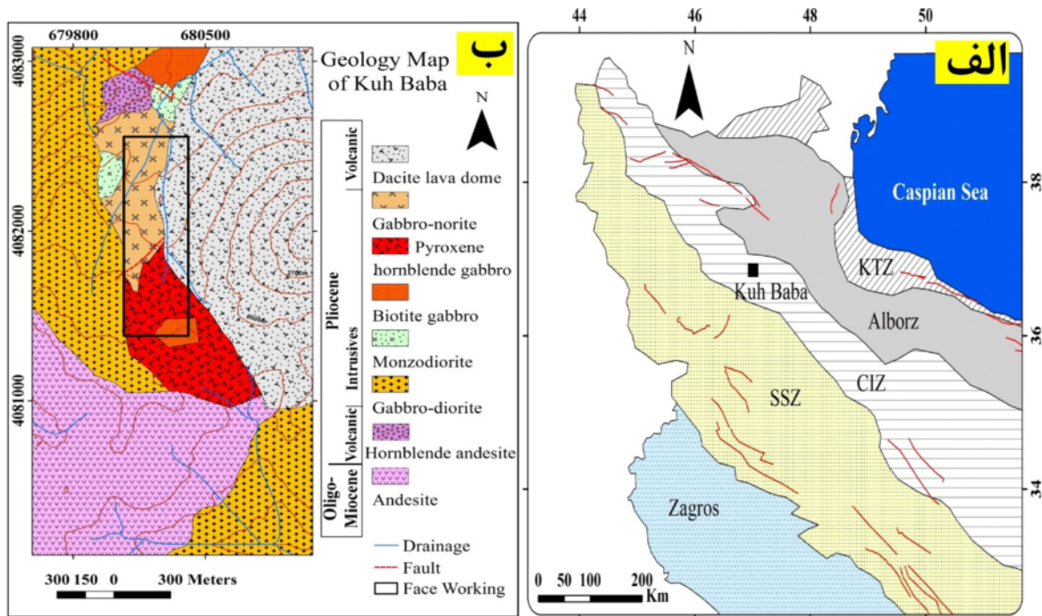
شکل ۱ الف) نقشه زمین‌ساختی ساده شده پهنه‌های رسوبی- ساختاری مختلف ایران و موقعیت کانسار آهن کوه‌بابا در آن (برگرفته از مراجع [۱۱، ۱۲] با اندکی تغییرات). علائم اختصاری به کار رفته در این شکل عبارتند از: SSZ = پهنه ماگمایی- دگرگونی سنندج- سیرجان، KTZ = پهنه ساختاری خزر- تالش- زیوه و CIZ = پهنه ایران مرکزی، ب) نقشه زمین‌شناسی کانسار آهن کوه‌بابا (برگرفته از مرجع [۹]). موقعیت سینه کار بر آن نشان داده شده است.
