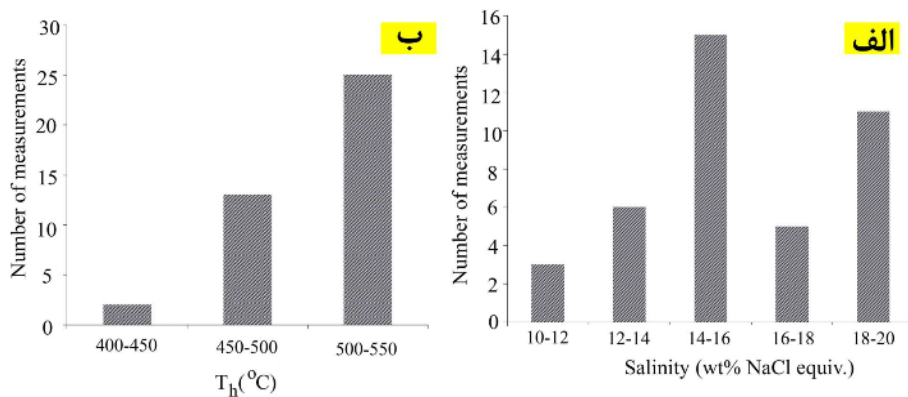
شکل ۸ (الف) نمودار دمای همگن شدگی مربوط به میانبرهای سیال در کانی سازی آهن کانسار کوهبابا با بیشترین فراوانی دمایی در گستره ۵۰۰ تا ۵۵۰ درجه سانتی گراد و (ب) نمودار شوری میانبرهای سیال بر حسب درصد وزنی با بیشترین فراوانی در گستره ۱۴ تا ۱۶ درصد وزنی معادل نمک طعام.
