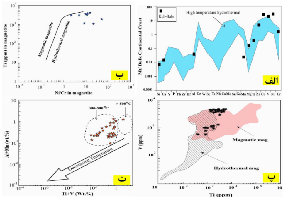
شکل ۶ (الف) نمودار چند عنصری [۲] که در آن گستره مگنتیت‌های گرمایی دما بالا نشان داده شده و اغلب نمونه‌های مورد بررسی در این گستره قرار می‌گیرند، (ب) نمودار دو متغیره Ti نسبت به Ni/Cr [۱۷] برای تفکیک محیط‌های ماگمایی از گرمایی، (پ) نمودار دو متغیره V نسبت به Ti [۱۹] برای تفکیک مگنتیت‌های ماگمایی از گرمایی. بر اساس نتایج EPMA، مگنتیت‌های کانسار آهن کوه‌بابا در گستره ماگمایی و گستره مشترک ماگمایی-گرمایی رسم می‌شوند و (ت) نمودار دو متغیره Ti+V نسبت به Al+Mn [۳] که نشان دهنده دمای تشکیل ۳۰۰ تا ۵۰۰ درجه سانتی‌گراد برای مگنتیت‌هاست.
