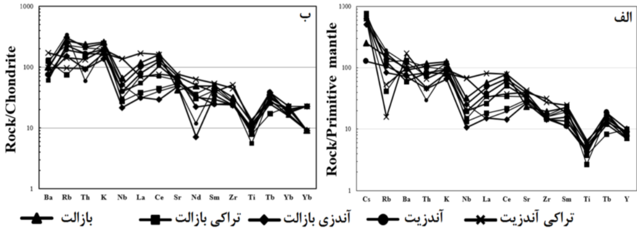
شکل ۷ نمودارهای عنکبوتی (چند عنصری) برای سنگ‌های آتشفشانی مورد بررسی بهنجار شده نسبت به الف ترکیب گوشته اولیه [۴۴]. و ب) کندریت [۴۸]. (بازالت مثلث، آندزیتی بازالت لوزی، تراکی بازالت مربع، آندزیت دایره و تراکی آندزیت ضربدر).
