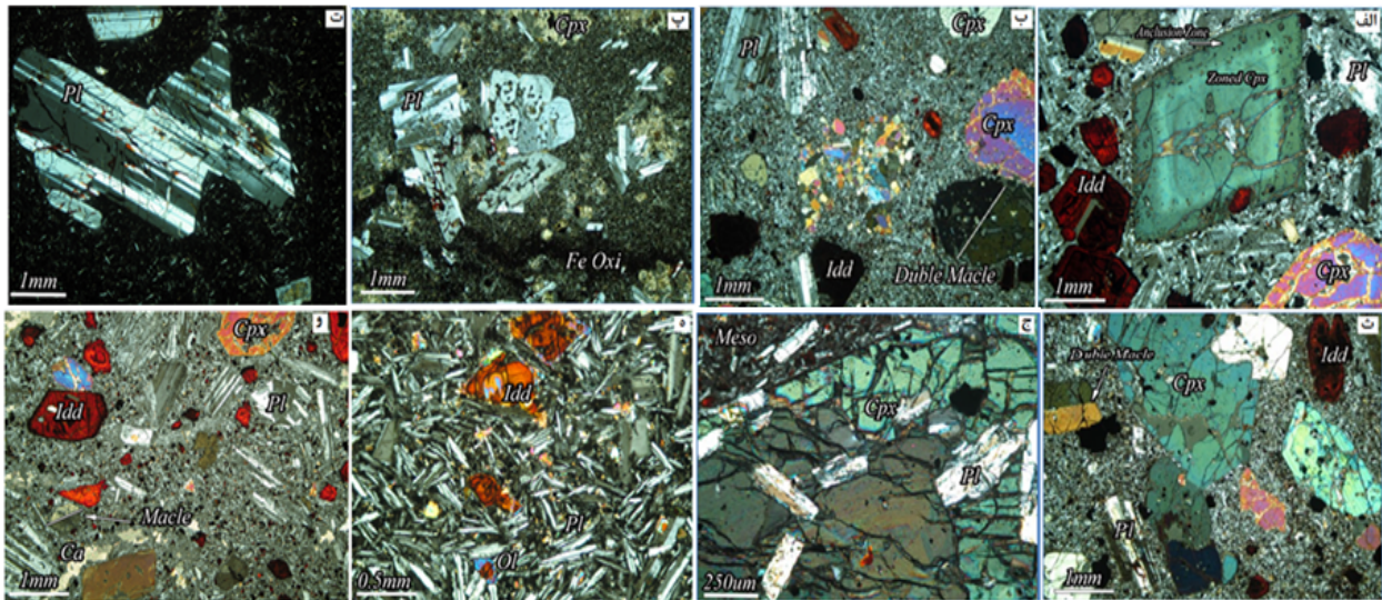
شکل ۳ تصاویر میکروسکوپی آندزیت و آندزیت بازالت‌ها: الف) بافت پورفیری؛ ب) بافت گلوپورفیری، پ) بافت غربالی در بلورهای پلاژیوکلاز، ت) خوردگی خلیج‌مانند در اطراف بلورهای پلاژیوکلاز، ث) ماکل دوتایی بلورهای کلینوپروکسن، ج) بافت غربالی، ه) بلورهای ایدینگزیتی شده الیون در خمیره‌ای ریزبلور، و) بافت میکرولیتی پورفیری. Pl: پلاژیوکلاز، Hb: هورنبلند، Cpx: کلینوپروکسن، Ol: الیون، Ca: کلسیت، Idd: ایدینگزیت، Fe Oxi: اکسید آهن [۳۲].
