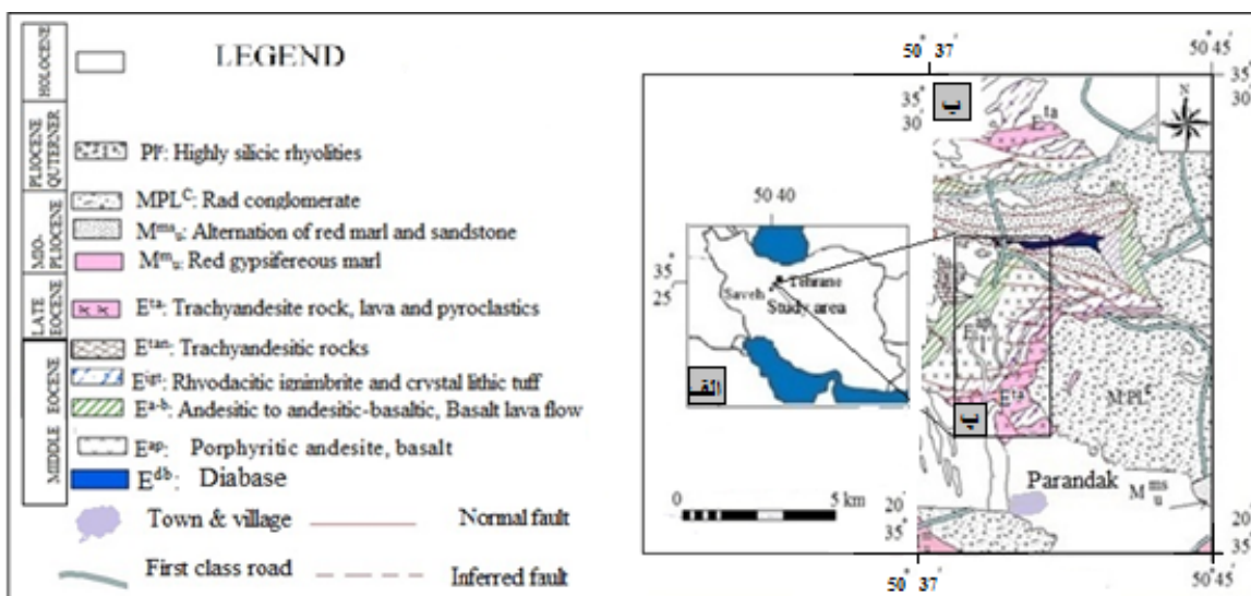
شکل ۱ الف- جایگاه منطقه مورد بررسی در نقشه ایران، ب- نقشه زمین شناسی منطقه مورد بررسی (برگرفته از نقشه زمین شناسی ۱:۱۰۰۰۰۰ زاویه (۱۳۸۴)، سازمان زمین شناسی کشور) و پ گستره نمونه برداری از زئولیت ها، سنگ میزبان آنها و واحدهای آتشفشانی و آذرآوری ائوسن میانی و بالایی.
