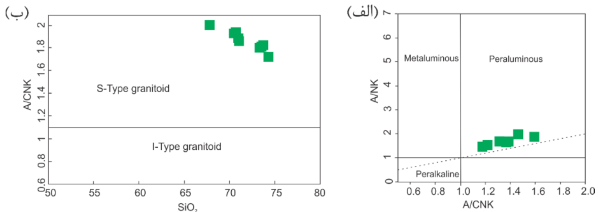
شکل ۶ الف) نمودار A/CNK نسبت به A/NK [۲۵] بخش روشن میگماتیت‌های بروجرد در گستره‌ی پرآلومین واقع شده‌اند. ب) نمودار SiO_2 نسبت به A/CNK [۳۶] که نمونه‌های روشن در گستره گرانیتهای نوع S قرار دارند.
