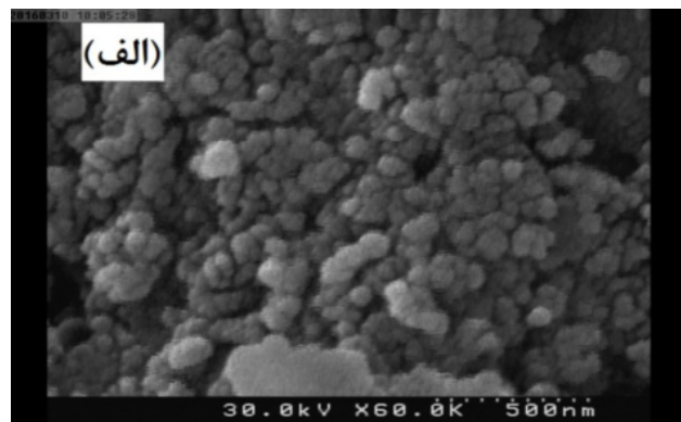
شکل ۲ تصاویر FESEM نمونه‌های (الف) خالص و (ب) با ۴٪ ناخالصی آلومینیوم.
