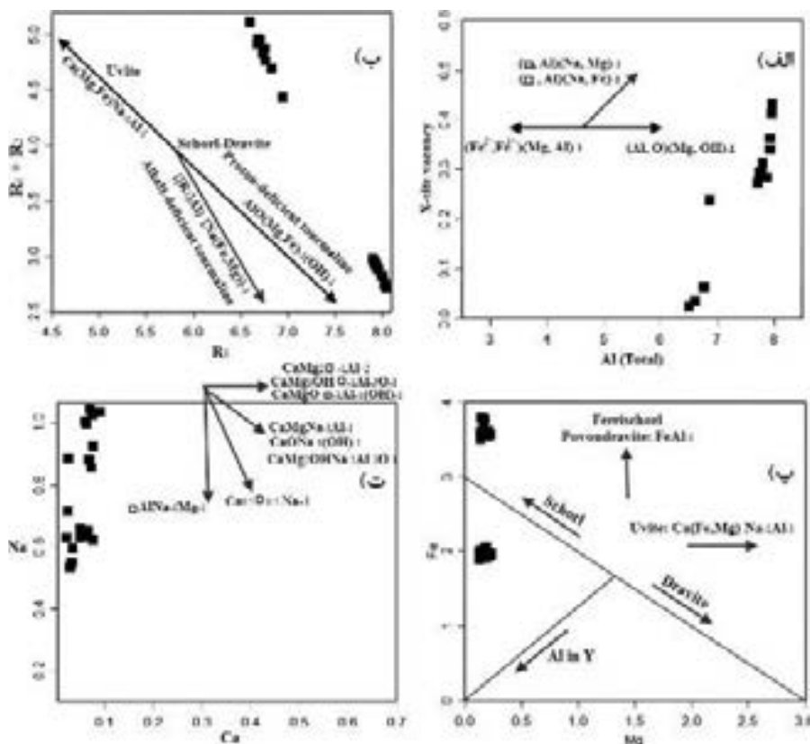
شکل ۵ الف) جایگاه تورمالین‌های مورد بررسی بر نمودار \text{Al}_{\text{Tot}} نسبت به X_{\text{vac}} [۲۲]. ب) جایگاه تورمالین‌های مورد بررسی بر نمودار R_2+R_3 نسبت به R_1 [۲۳] که R_3=\text{Al}+1.33\text{Ti} ، R_2=\text{Fe}+\text{Mg}+\text{Mn} ، R_1=\text{Ca}+\text{Na} که ترکیب آرمانی شورل-دراویت نشان دهنده‌ی جانشینی‌های یوویت (پیکان بالایی) و جانشینی‌های تورمالین‌های ناقص از نظر قلیایی و پروتون‌زدایی (پیکان‌های پایینی) هستند، پ) جایگاه تورمالین‌های مورد بررسی بر نمودار Fe نسبت به Mg [۲۴]. ت) جایگاه تورمالین‌های مورد بررسی بر نمودار Na نسبت به Ca [۲۵].
