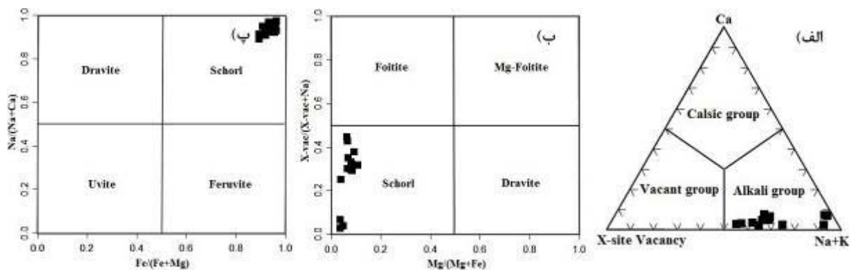
شکل ۴ الف) نمودار مثلثی Ca-(X-vac)-Na+(K) [۱۶]، و جایگاه نمونه‌های مورد بررسی بر آن، ب) جایگاه تورمالین-های مورد بررسی بر نمودار vac/(X-vac+Na) نسبت به Mg/(Mg+Fe) [۱۹] و ب) جایگاه تورمالین‌ها بر نمودار Na/(Na+Ca) نسبت به Fe/(Fe+Mg) [۲۰].
