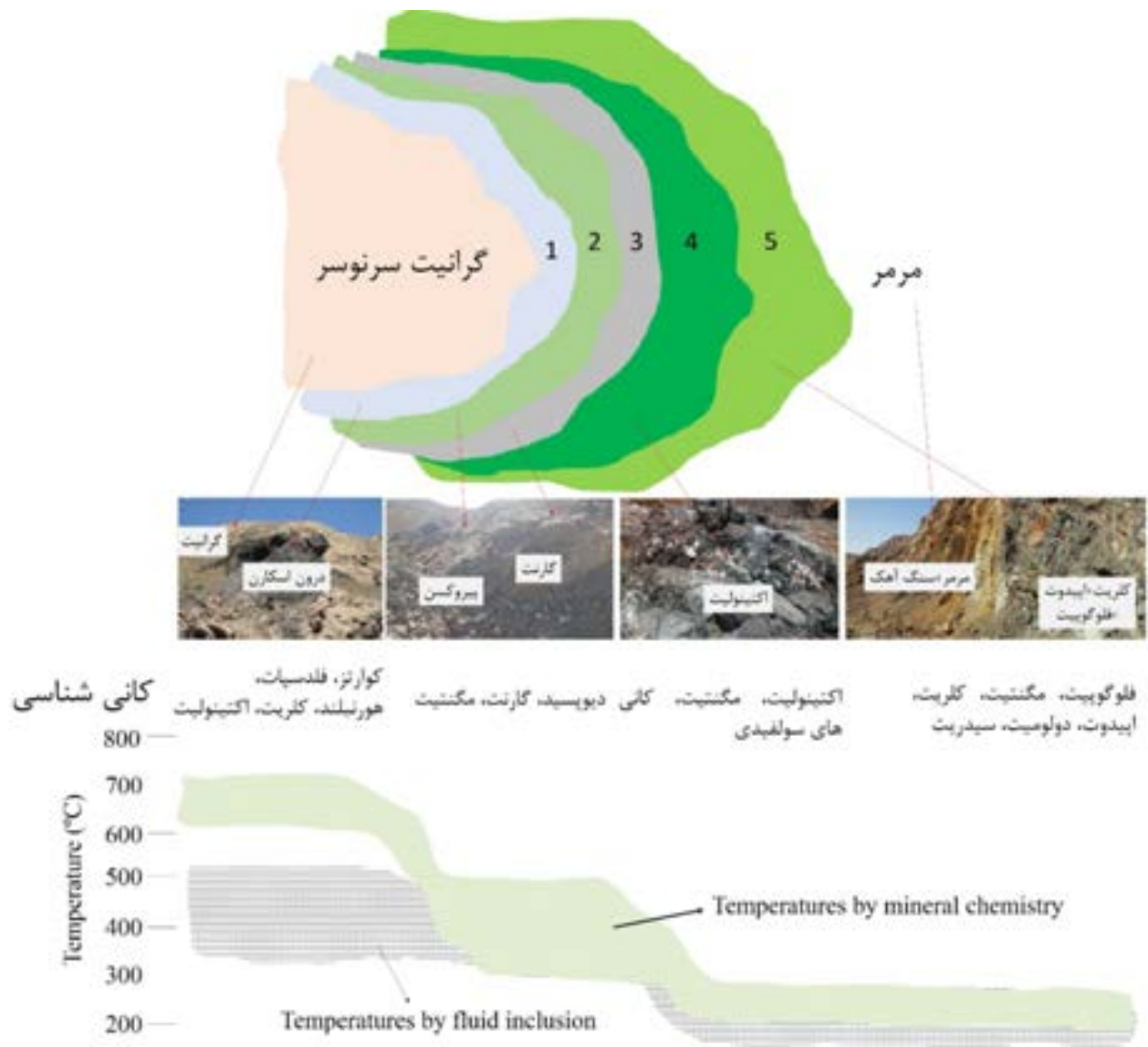
شکل ۸ طرحواره بدون مقیاس از پهنه‌های اسکارنی پیرامون گرانیت سرنوسر همراه با کانی‌شناسی غالب در هر پهنه و دماهای بدست آمده بر اساس ترکیب شیمیایی کانی‌ها و میانبراهای سیال که روند کاهش دما از درون‌اسکارن، پهنه پیشرونده به سمت پهنه پسرونده مشخص است.
