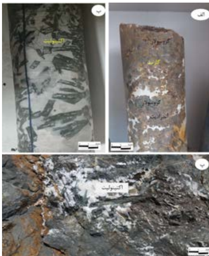
شکل ۴ الف) درشت‌بلورهای آندرادیت (قهوه‌ای رنگ) و گروسولار (سبزرنگ) در اسکارن پیشرونده (پهنه گارنت اسکارن)، ب و پ) درشت‌بلورهای خودشکل اکتینولیت در اسکارن پسروده.
