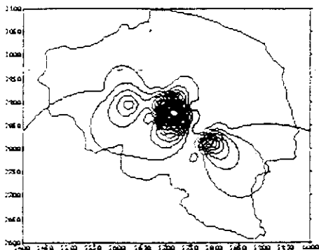
مدل کریجینگ
