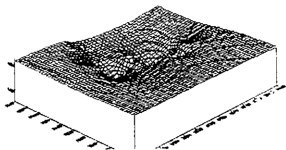
مدل کریجینگ
