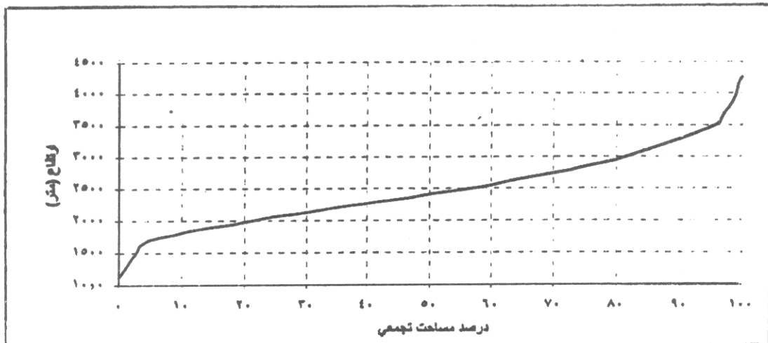
شکل ۱- منحنی تغییرات سطح با ارتفاع در حوضه آبریز طالقان (منحنی هیسومتریک)
