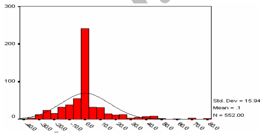
شکل ۱۱- نمودار هیستوگرام فراوانی باقیمانده های مدل سری زمانی بارش ماهانه بیرجند
