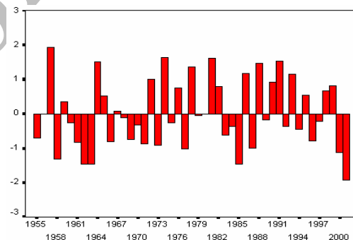
نمره Z استاندارد فصل زمستان ایستگاه
