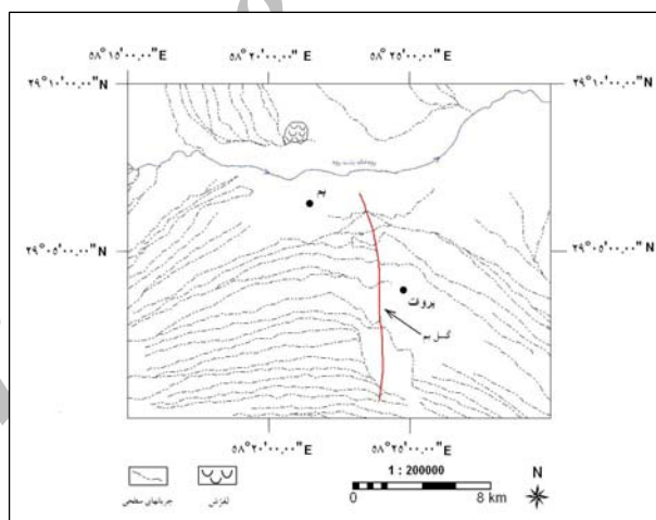
شکل ۱۴: انحرافات به وجود آمده در شبکه هیدروگرافی منطقه بر اثر فعالیت گسل در بخش غربی گسل به خوبی قابل مشاهده است. مأخذ: سازمان جغرافیایی نیروهای مسلح، نقشه توپوگرافی ۱:۵۰۰۰۰ منطقه بم
